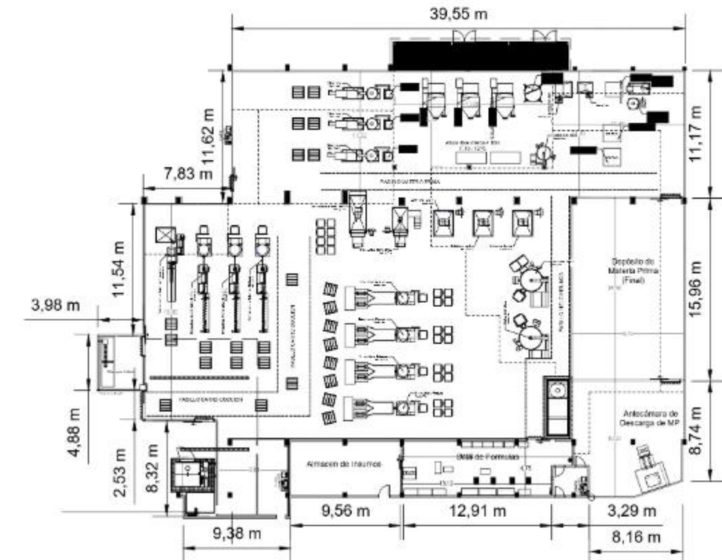
LAYOUT — SALA DE EMBUTIDOS
