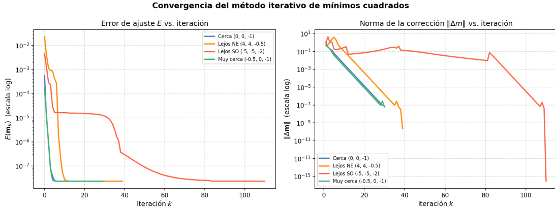
Figura 9: Izquierda: evolución de E(\mathbf{m}_k) en escala logarítmica para los cuatro puntos de partida. Derecha: norma \|\Delta \mathbf{m}\| por iteración. Todos los inicios convergen al mismo nivel de error, demostrando robustez del método de Levenberg–Marquardt.
