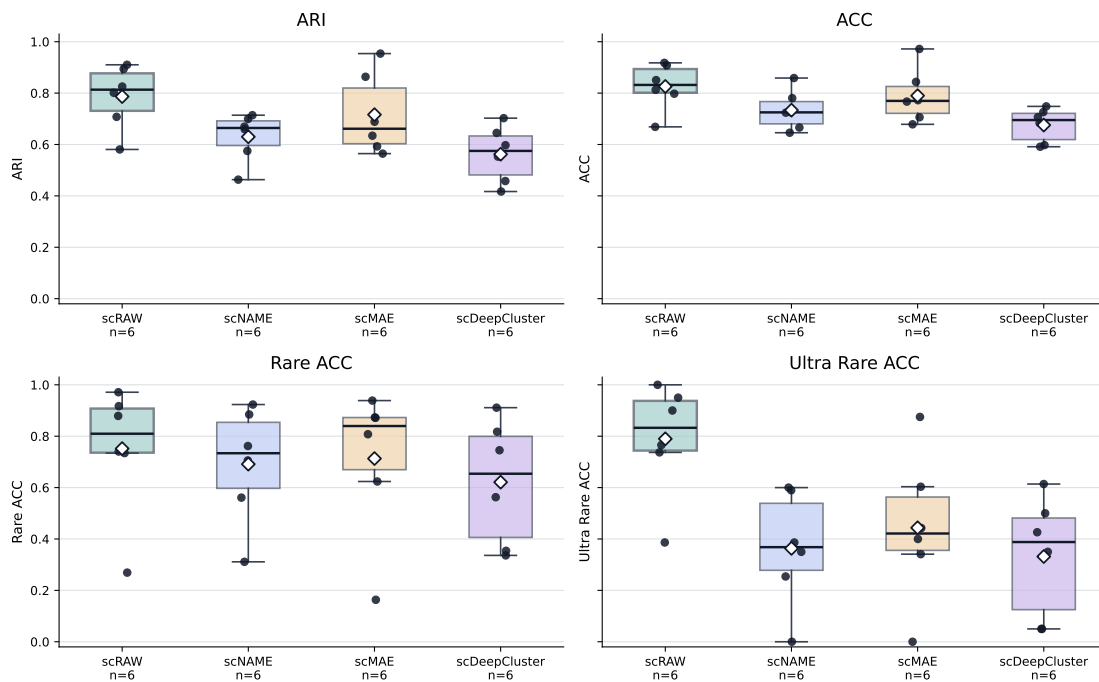
FIGURE 12 – Distribution des performances inductives pour ARI, ACC, RareACC et Ultra-RareACC. Les boîtes représentent la distribution des moyennes par jeu de données et split inductif pour chaque algorithme testé. Chaque point noir correspond à la moyenne d'un jeu de données et les losanges blancs indiquent la moyenne globale de l'algorithme.
