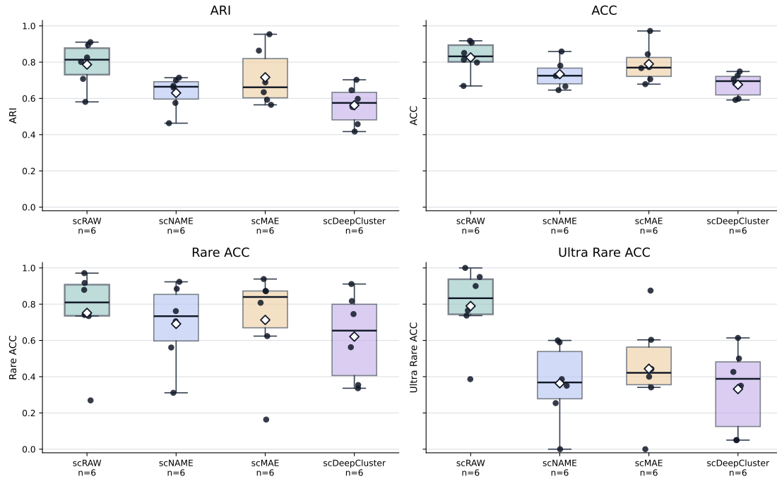
FIGURE 6 – Comparaison inductive de scRAW avec scNAME, scMAE et scDeepCluster sur six jeux de données. Chaque boîte représente la distribution des moyennes par jeu de données, et chaque point correspond à un jeu de données. Les losanges indiquent la moyenne globale de l’algorithme pour la métrique considérée.
