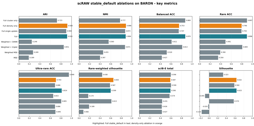
FIGURE 13 – Comparaison graphique des performances des variantes d’ablation de scRAW pour les métriques de clustering global (ARI, NMI, ACC), la détection des classes rares (RareACC, UltraRareACC) et le score d’intégration de batch (scIB-E).
