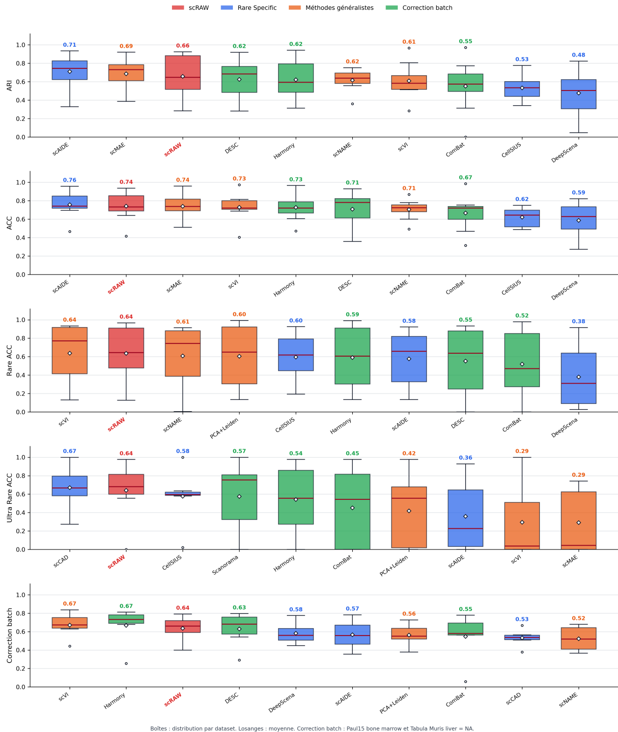
FIGURE 4 – Distribution des performances sur les huit jeux de données communs. scRAW est comparé aux trois meilleures méthodes de chaque famille pour chaque métrique. Les boîtes résument les scores par jeu de données ; les points noirs indiquent les valeurs individuelles et le losange blanc la moyenne.
