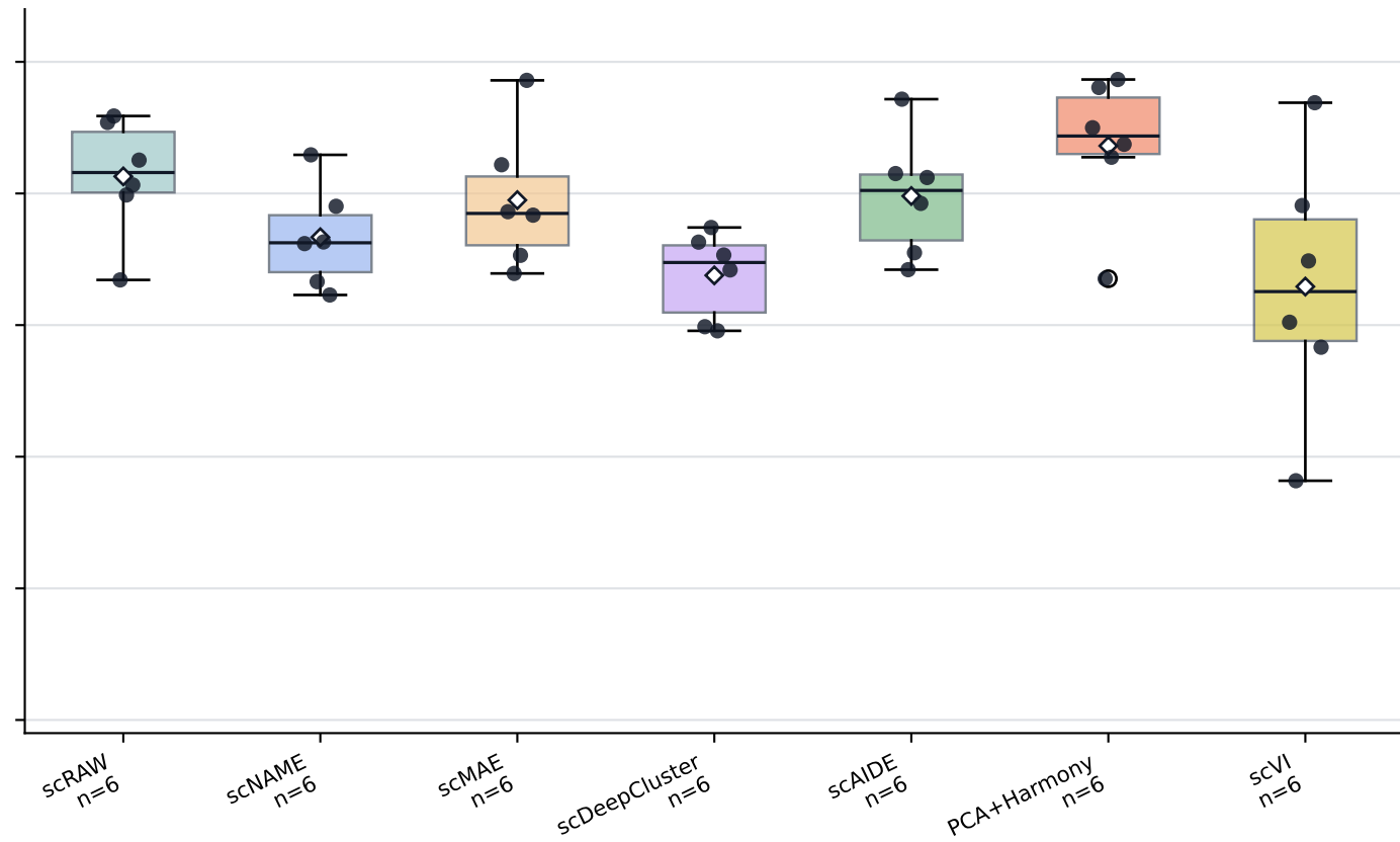
ACC
