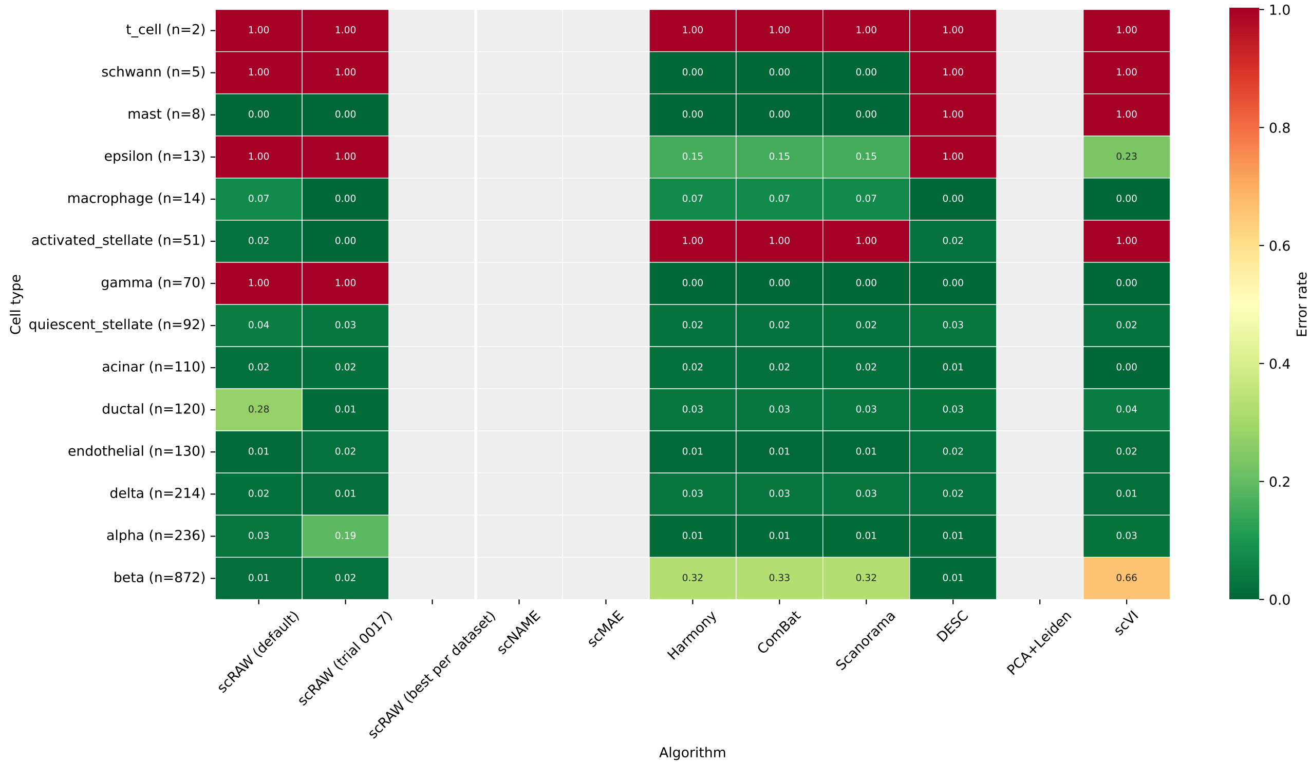
SCIB Human Pancreas 1 - erreur de prediction par type cellulaire
