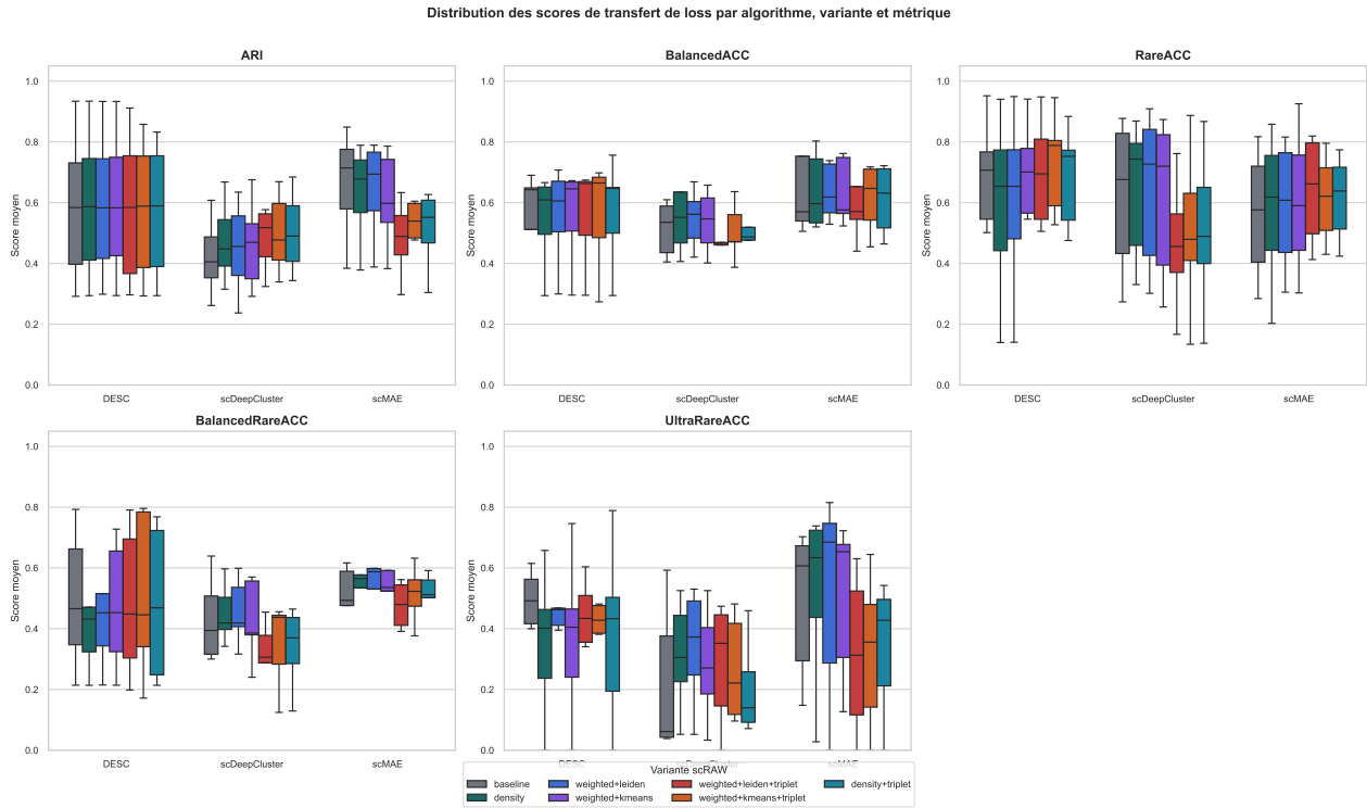
FIGURE 12 – Distribution des scores pour toutes les configurations testées lors du transfert de la loss pondérée \mathcal{L}_{\text{recon}, \text{ponderee}} de scRAW sur 5 jeux de données. Les cinq panneaux correspondent aux métriques ARI, BalancedACC, RareACC, UltraRareACC et BalancedRareACC. Les boîtes représentent la distribution des scores moyens sur les 5 jeux de données communs.
