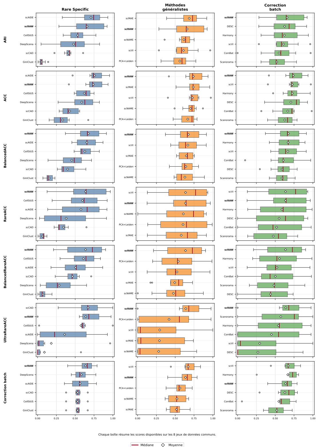
FIGURE 10 – Résultats complets par famille sur les 8 jeux de données communs. Les boîtes résument la distribution des scores pour ces 8 jeux de données par méthode ; le losange blanc indique la moyenne ; les jeux sans classe ultra-rare ne contribuent pas à l'UltraRareACC. scRAW est ajouté comme repère dans chaque famille.
