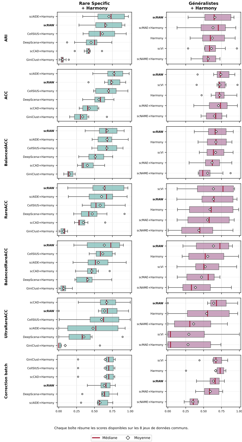
FIGURE 11 – Résultats complémentaires avec Harmony sur les 8 jeux de données communs. Les boîtes résument la distribution des scores pour ces 8 jeux de données par méthode ; le losange blanc indique la moyenne. Les méthodes Rare Specific +Harmony sont indiquées à titre exploratoire, car cette association n'est pas documentée comme usage standard par les auteurs. Pour les méthodes de deep learning généralistes, Harmony est appliqué sur l'espace latent avant le clustering final. La ligne Harmony correspond au pipeline PCA+Harmony avant clustering ; scVI est conservé comme méthode native intégrant l'information de batch.
