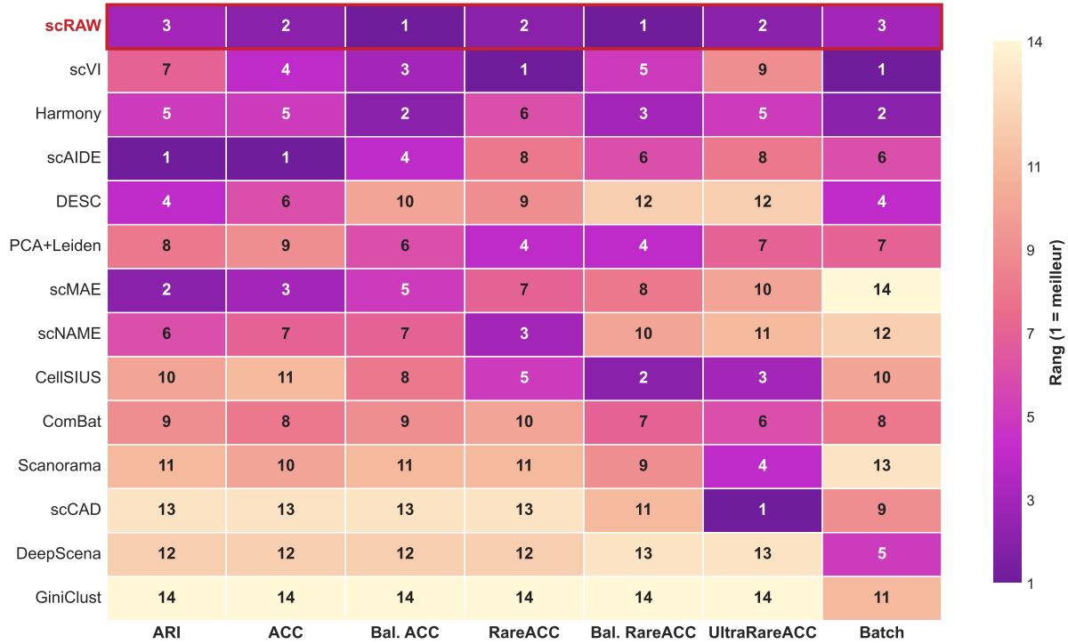
FIGURE 5 – Matrice de rangs des algorithmes selon les métriques moyennes sur le jeu commun (8 jeux de données). Les lignes correspondent aux méthodes et les colonnes aux métriques affichées dans la section : ARI, ACC, BalancedACC, RareACC, BalancedRareACC, UltraRareACC et correction de batch. Le rang 1 correspond à la meilleure moyenne pour une métrique donnée. Les cases suivent un dégradé du violet (meilleur rang) au jaune clair (rang moins favorable). La matrice ne contient pas de colonne de score moyen ni de rang global, afin de faire apparaître directement les compromis métrique par métrique.
