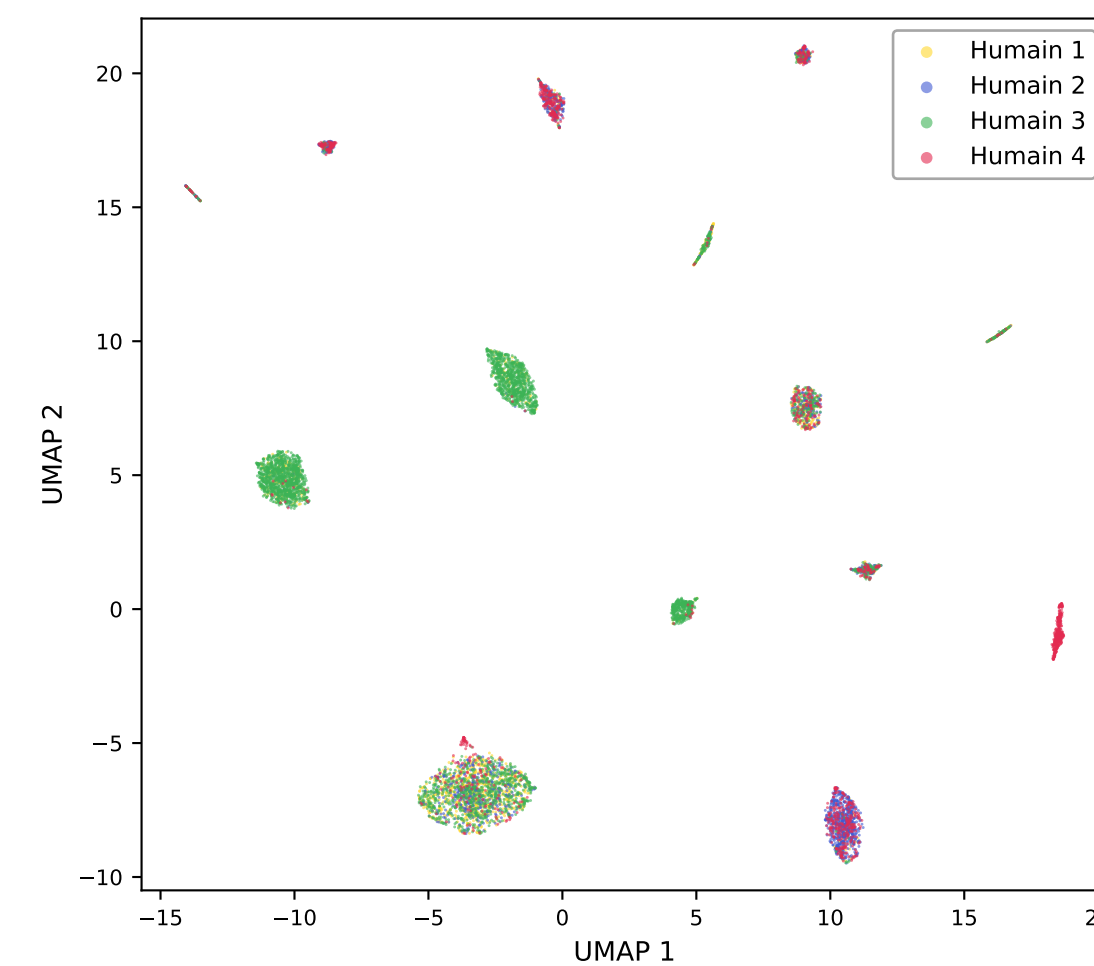
scNAME
