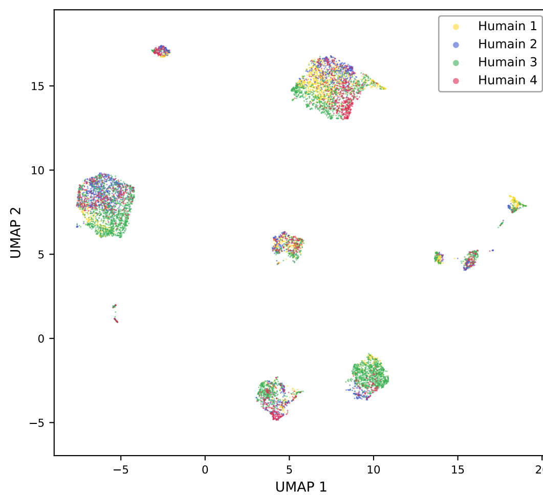
scVI
