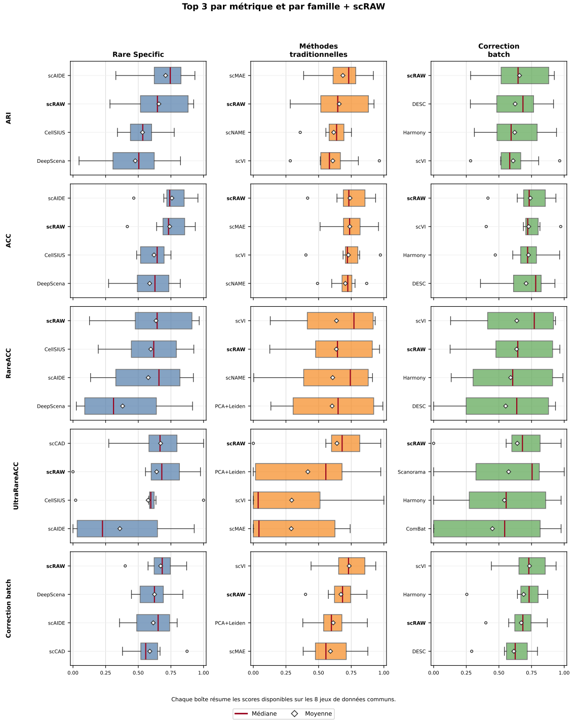
FIGURE 5 – Distribution des performances sur les huit jeux de données communs, par famille de méthodes. Chaque boîte correspond aux scores disponibles sur les jeux de données ; pour l'UltraRareACC, les jeux sans classe ultra-rare ne contribuent pas à la distribution. Les méthodes sont ordonnées par moyenne croissante dans chaque sous-panneau. Chaque sous-panneau affiche scRAW et les trois meilleures méthodes de la famille pour la métrique considérée.
