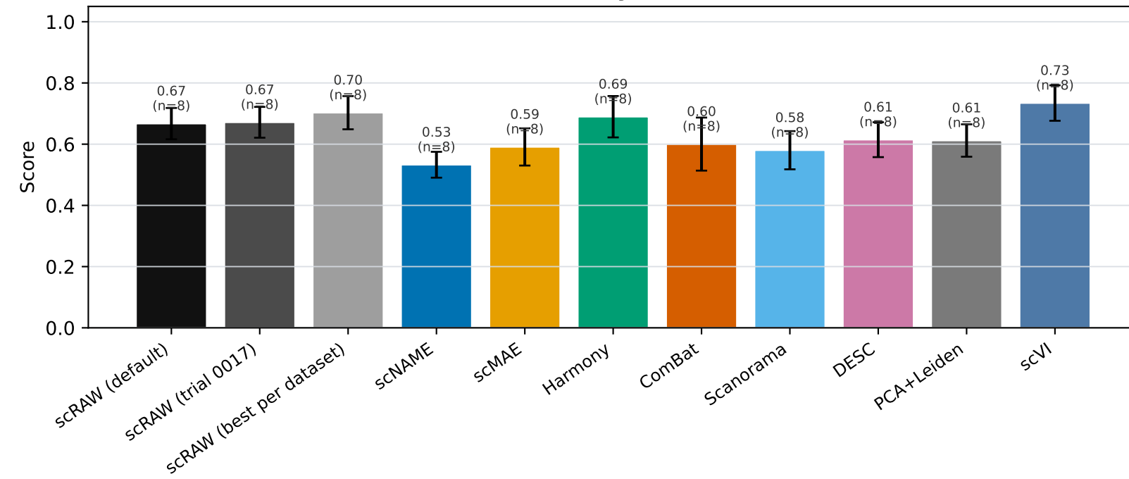
Batch correction - moyenne sur 8 datasets
