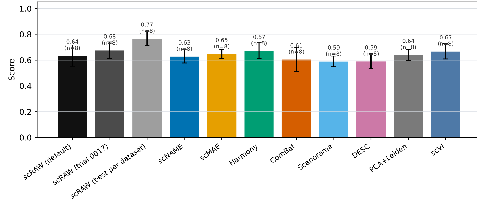
Batch correction - moyenne sur 8 datasets
