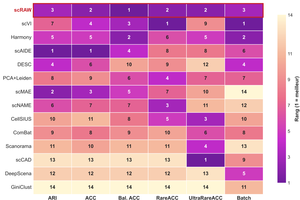
FIGURE 5 – Matrice de rangs des algorithmes selon les métriques moyennes sur le jeu commun common-8 . Les lignes correspondent aux méthodes et les colonnes aux métriques affichées dans la section : ARI, ACC, BalancedACC, RareACC, UltraRareACC et correction de batch. Le rang 1 correspond à la meilleure moyenne pour une métrique donnée. Les cases suivent un dégradé du violet (meilleur rang) au jaune clair (rang moins favorable). La matrice ne contient pas de colonne de score moyen ni de rang global, afin de faire apparaître directement les compromis métrique par métrique.
