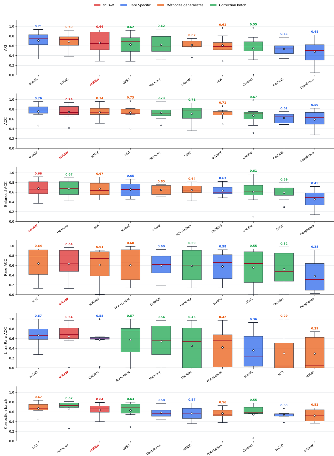
FIGURE 4 – Distribution des performances sur les huit jeux de données communs. scRAW est comparé aux trois meilleures méthodes de chaque famille pour chaque métrique. Les boîtes résument les scores par jeu de données ; les points noirs indiquent les valeurs individuelles et le losange blanc la moyenne.
