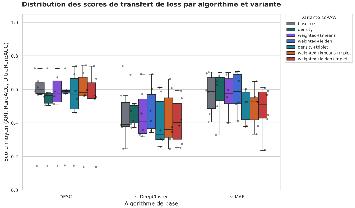
FIGURE 11 – Distribution des scores pour toutes les configurations testées lors du transfert de la loss pondérée \mathcal{L}_{\text{recon,ponderee}} de scRAW. Les boîtes représentent la distribution des scores moyens (moyenne de l'ARI, de la RareACC et de l'UltraRareACC) sur l'ensemble des jeux de données.
