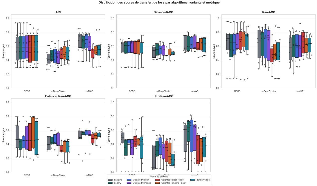
FIGURE 12 – Distribution des scores pour toutes les configurations testées lors du transfert de la loss pondérée \mathcal{L}_{\text{recon, ponderee}} de scRAW sur 8 jeux de données. Les cinq panneaux correspondent aux métriques ARI, BalancedACC, RareACC, UltraRareACC et BalancedRareACC. Les boîtes représentent la distribution des scores moyens sur les 8 jeux de données communs, et les points noirs indiquent les valeurs par jeu de données.
