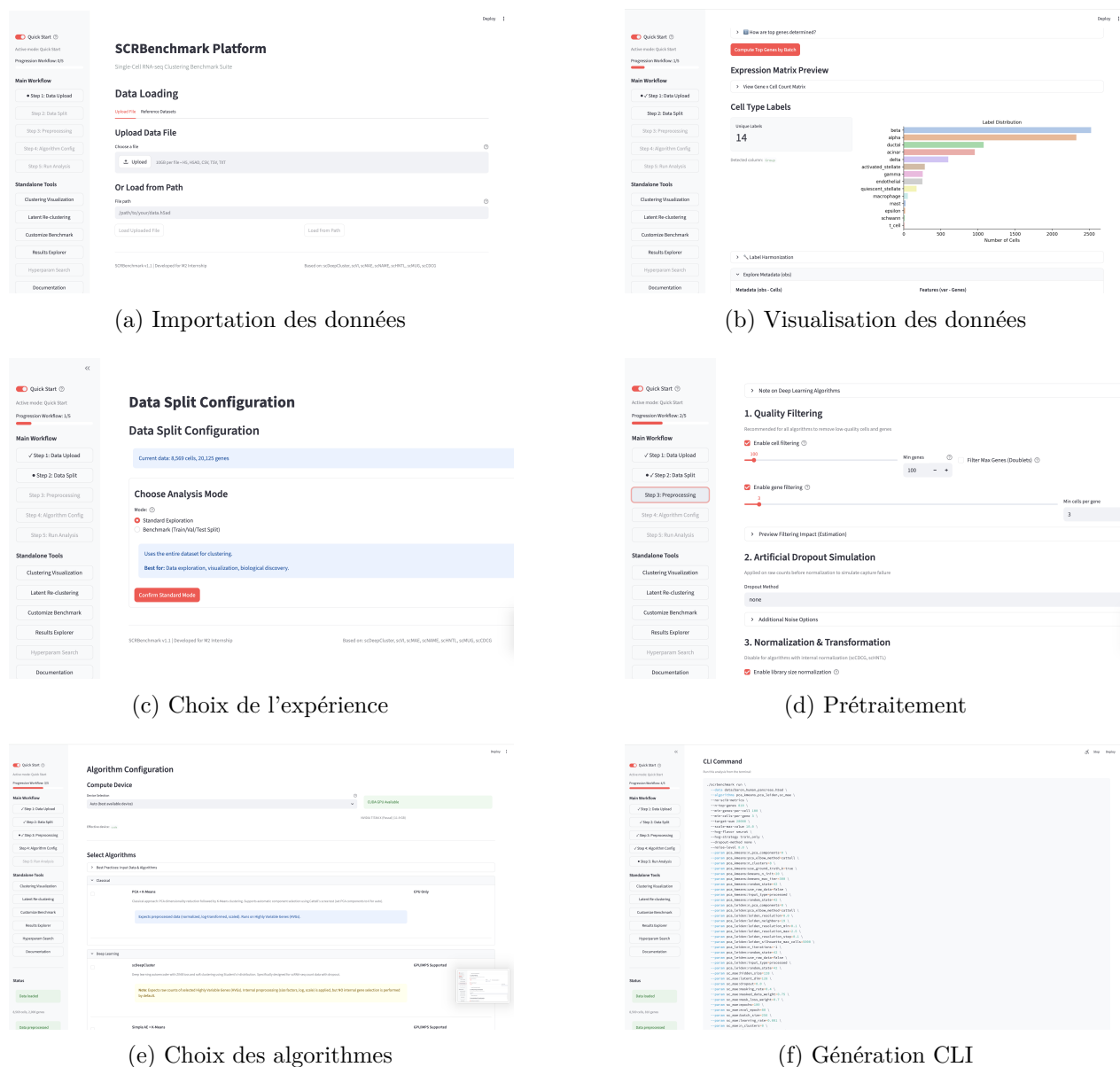
FIGURE 19 – Aperçu des différentes étapes de l’interface Streamlit de SCRBenchmark (1 re partie : configuration et préparation).
