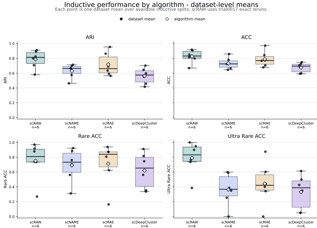
FIGURE 6 – Comparaison inductive de scRAW avec scNAME, scMAE et scDeepCluster sur six jeux de données. Chaque boîte représente la distribution des moyennes par jeu de données, et chaque point correspond à un jeu de données. Les losanges indiquent la moyenne globale de l’algorithme pour la métrique considérée.
