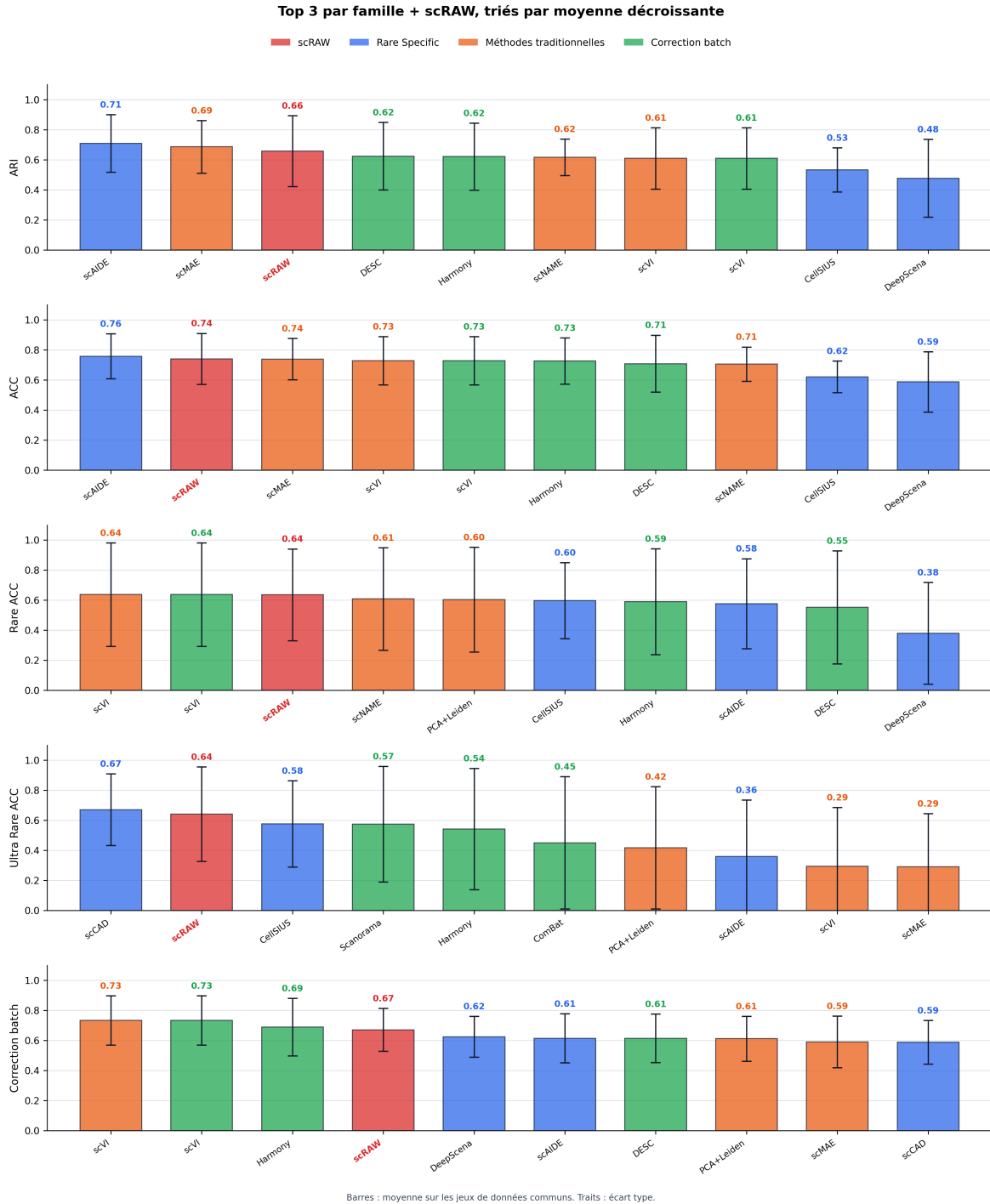
FIGURE 4 – Performances moyennes sur les huit jeux de données communs pour scRAW et le top 3 de chaque famille de méthodes. Chaque panneau correspond à une métrique (de haut en bas : ARI, ACC, Rare ACC, Ultra Rare ACC, Correction batch). Les couleurs identifient les familles de méthodes : scRAW (rouge), Rare Specific (bleu), Méthodes traditionnelles (orange) et Correction batch (vert). Pour chaque métrique, les méthodes représentées (scRAW et les trois meilleures de chaque famille) sont triées globalement par moyenne décroissante (meilleure à gauche). Les barres représentent le score moyen sur les jeux de données communs (la valeur est indiquée au-dessus de chaque barre), et les barres d'erreur représentent l'écart type ; pour l'Ultra Rare ACC, les jeux sans cellules ultra-rares ne contribuent pas au calcul.
