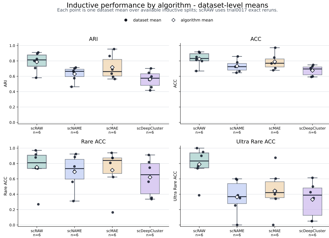
FIGURE 12 – Distribution des performances inductives pour ARI, ACC, RareACC et Ultra-RareACC. Les boîtes représentent la distribution des moyennes par jeu de données et split inductif pour chaque algorithme testé.
