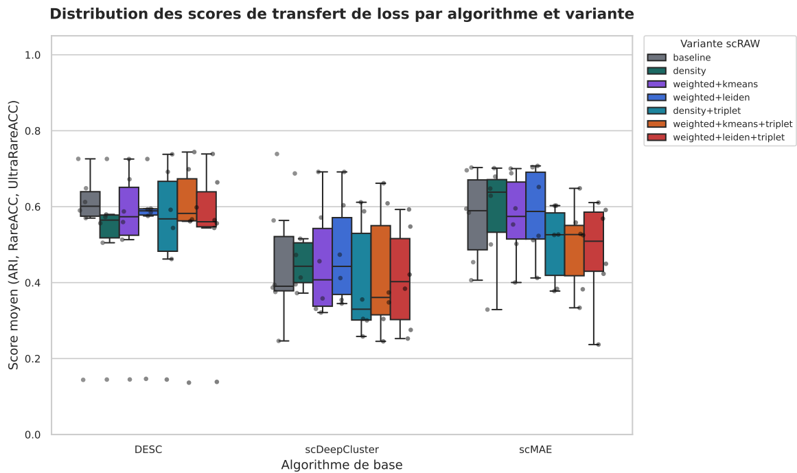
FIGURE 11 – Distribution des scores pour toutes les configurations testées lors du transfert de la loss pondérée scRAW. Les boîtes représentent la distribution des scores moyens (moyenne de l'ARI, de la RareACC et de l'UltraRareACC) sur l'ensemble des jeux de données.
