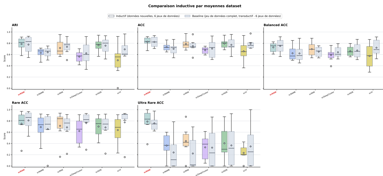
FIGURE 13 – Distribution des performances inductives pour ARI, ACC, Balanced ACC, RareACC et UltraRareACC sur 6 jeux de données. Les boîtes représentent la distribution des moyennes par jeu de données et split inductif pour chaque algorithme testé ; les losanges blancs indiquent la moyenne globale de l'algorithme.
