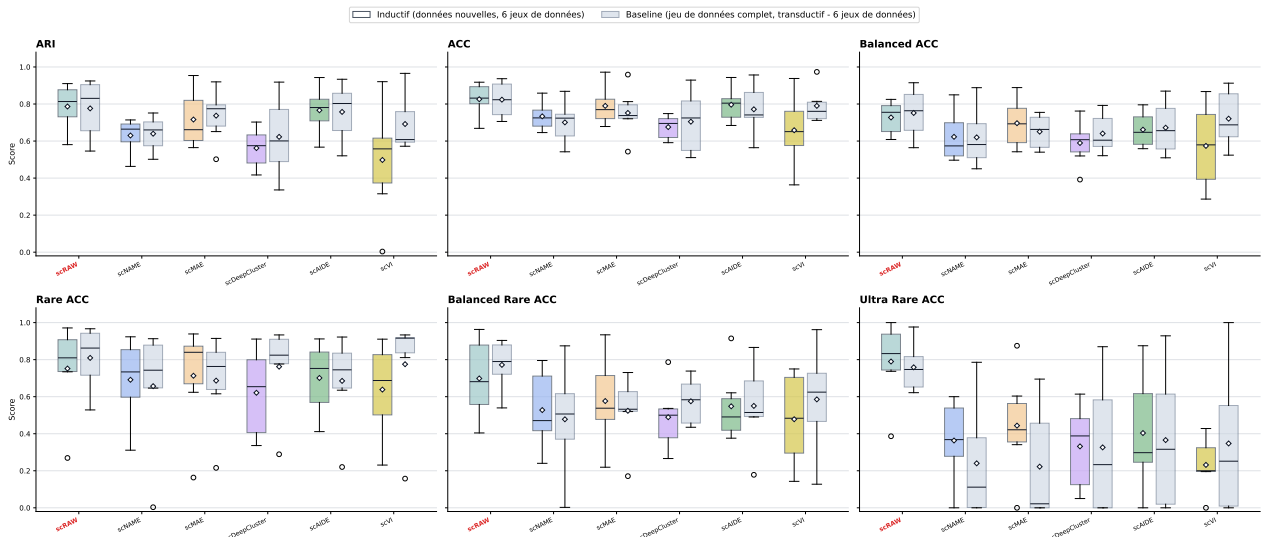
FIGURE 7 – Comparaison des performances en mode inductif (boîtes colorées, sur données tests non vues) et transductif (boîtes grisées, baseline entraînée sur tout le jeu de données et moyennée) pour 6 algorithmes sur les 6 jeux de données. Chaque boîte représente la distribution des moyennes par jeu de données. Les losanges indiquent la moyenne globale pour chaque métrique.
