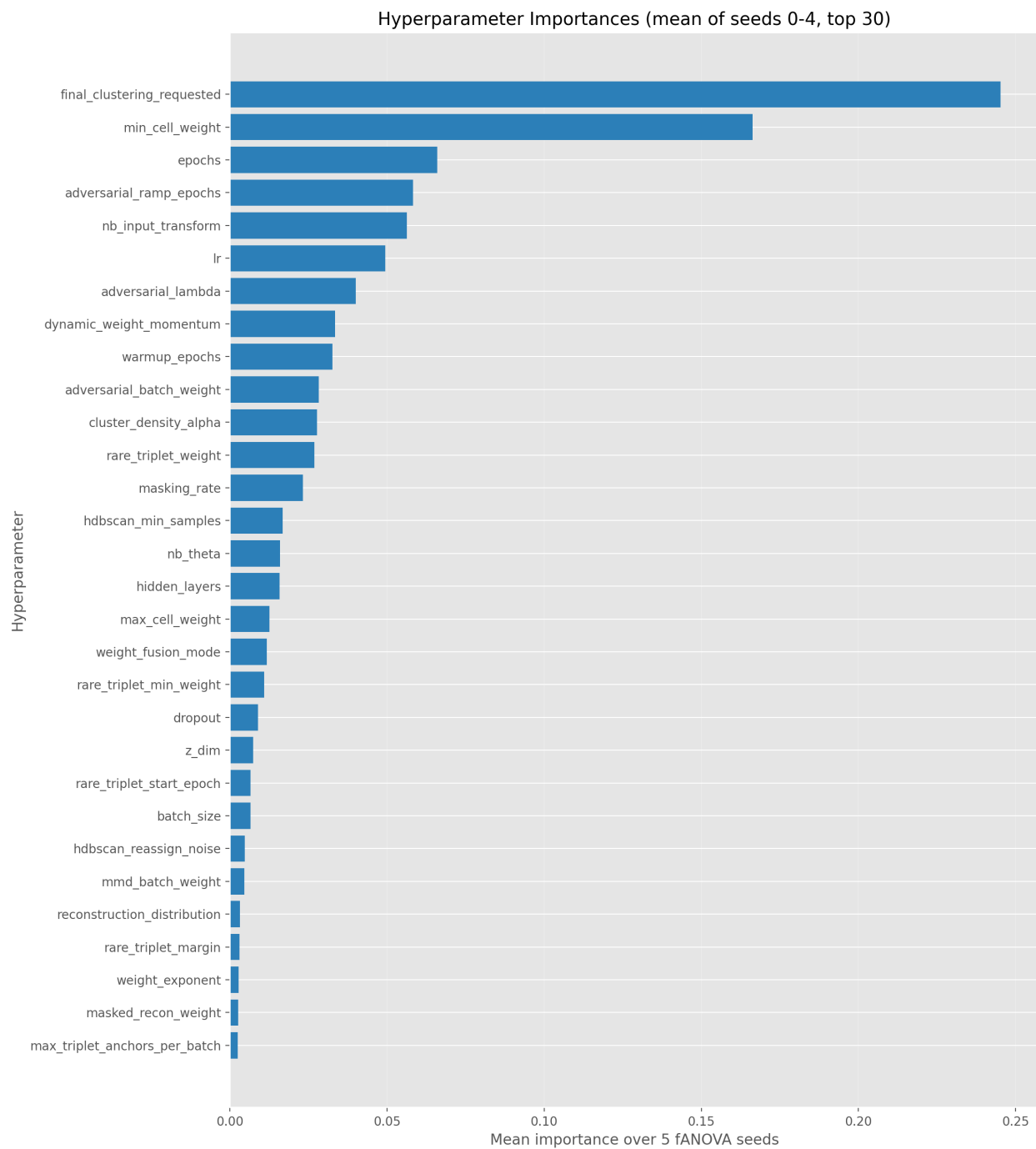
FIGURE 16 – Importance des hyperparamètres pour la campagne 2 (généraliste sur 8 jeux de données).
