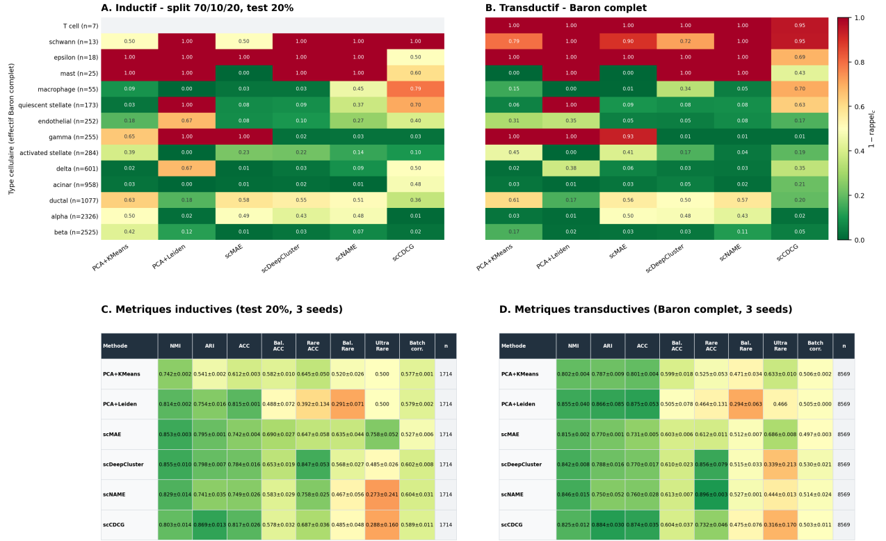
FIGURE 2 – Panel de résultats sur le jeu de données Baron. A–B : valeur 1 - \text{rappel}_c par type cellulaire et par méthode, en mode inductif sur le test du split stratifié 70/10/20 et en mode transductif sur le jeu complet, avec \text{rappel}_c = \text{TP}_c / (\text{TP}_c + \text{FN}_c) après appariement hongrois. C–D : métriques globales associées. Les deux cadres sont moyennés sur trois seeds et utilisent le prétraitement du protocole de comparaison. Pour PCA+Leiden, la résolution est sélectionnée par recherche de silhouette et le nombre de clusters n’est pas fixé à 14.
