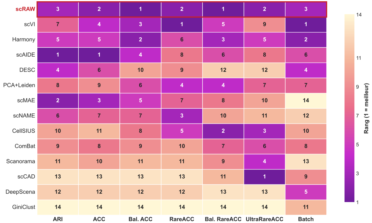
FIGURE 5 – Matrice de rangs des algorithmes selon les métriques moyennes sur le jeu commun (8 jeux de données) . Les lignes correspondent aux méthodes et les colonnes aux métriques affichées dans la section : ARI, ACC, BalancedACC, RareACC, BalancedRareACC, UltraRareACC et correction de batch. Le rang 1 correspond à la meilleure moyenne pour une métrique donnée. Les cases suivent un dégradé du violet (meilleur rang) au jaune clair (rang moins favorable). La matrice ne contient pas de colonne de score moyen ni de rang global, afin de faire apparaître directement les compromis métrique par métrique.
