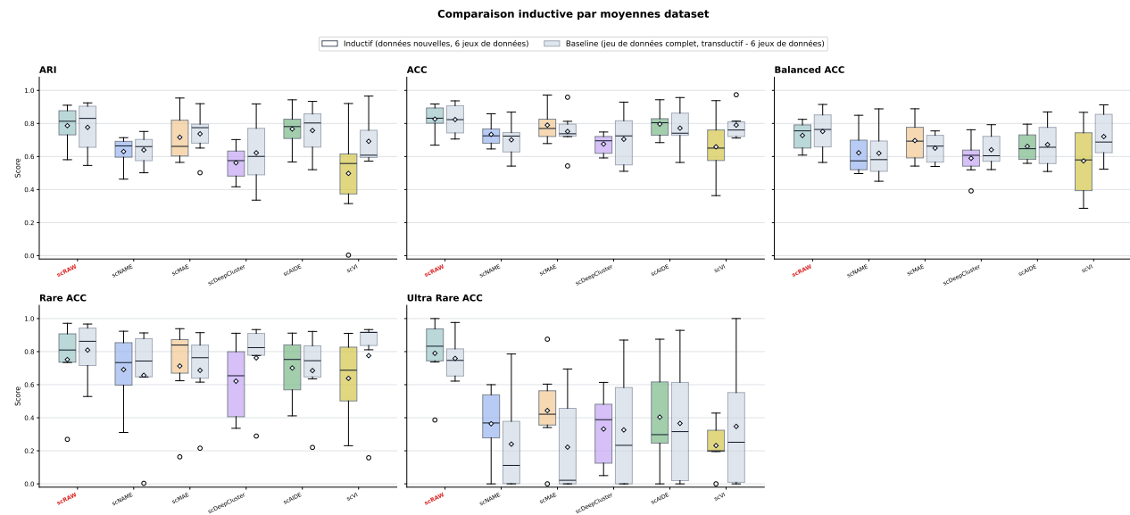
FIGURE 13 – Distribution des performances inductives pour ARI, ACC, Balanced ACC, RareACC et UltraRareACC sur 6 jeux de données. Les boîtes représentent la distribution des moyennes par jeu de données et split inductif pour chaque algorithme testé. Chaque point noir correspond à la moyenne d'un des 6 jeux de données et les losanges blancs indiquent la moyenne globale de l'algorithme.
