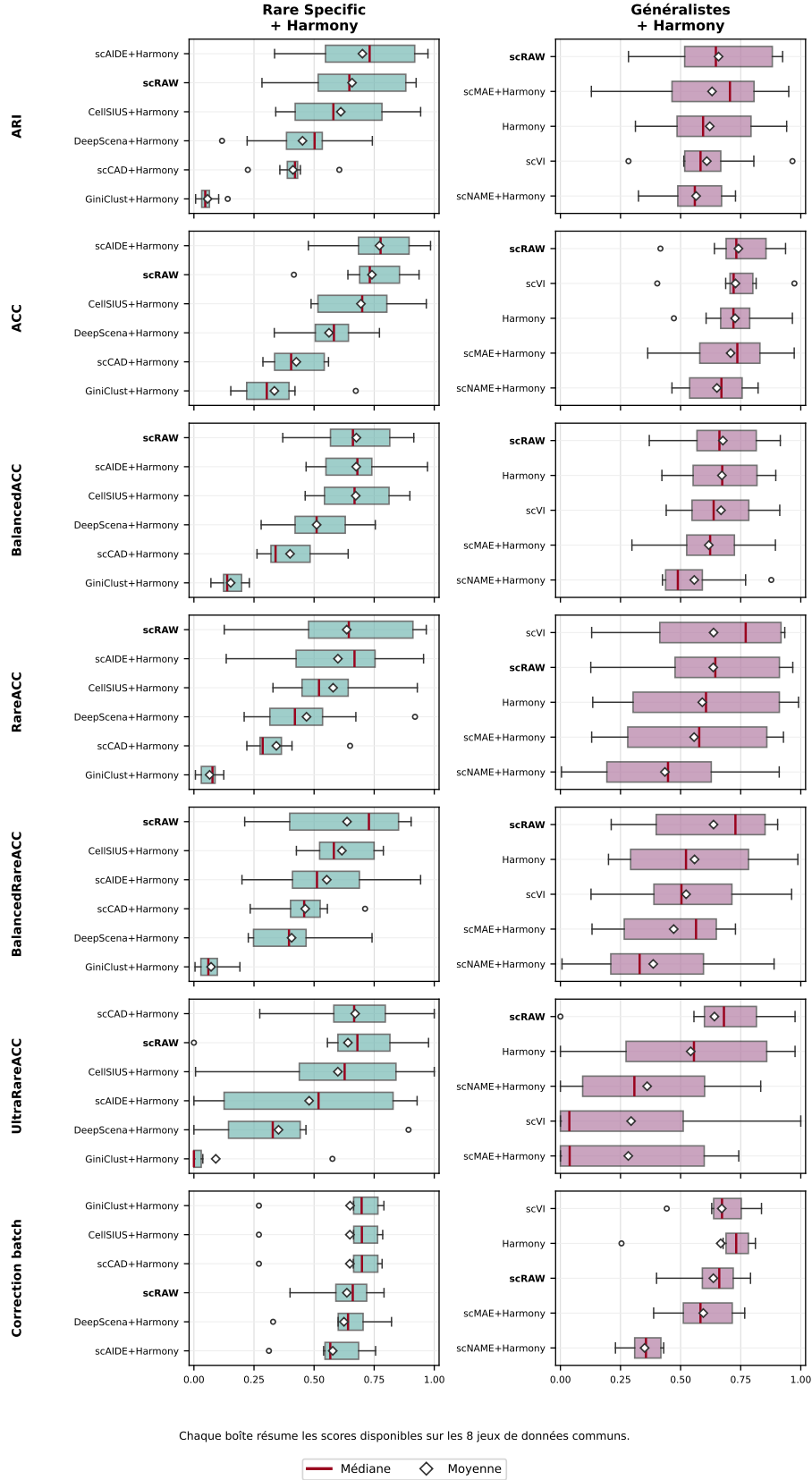
FIGURE 11 – Résultats complémentaires avec Harmony sur les 8 jeux de données communs. Les méthodes Rare Specific +Harmony sont indiquées à titre exploratoire, car cette association n'est pas documentée comme usage standard par les auteurs. Pour les méthodes de deep learning généralistes, Harmony est appliqué sur l'espace latent avant le clustering final. La ligne Harmony correspond au pipeline PCA+Harmony avant clustering; scVI est conservé comme méthode native intégrant l'information de batch.
