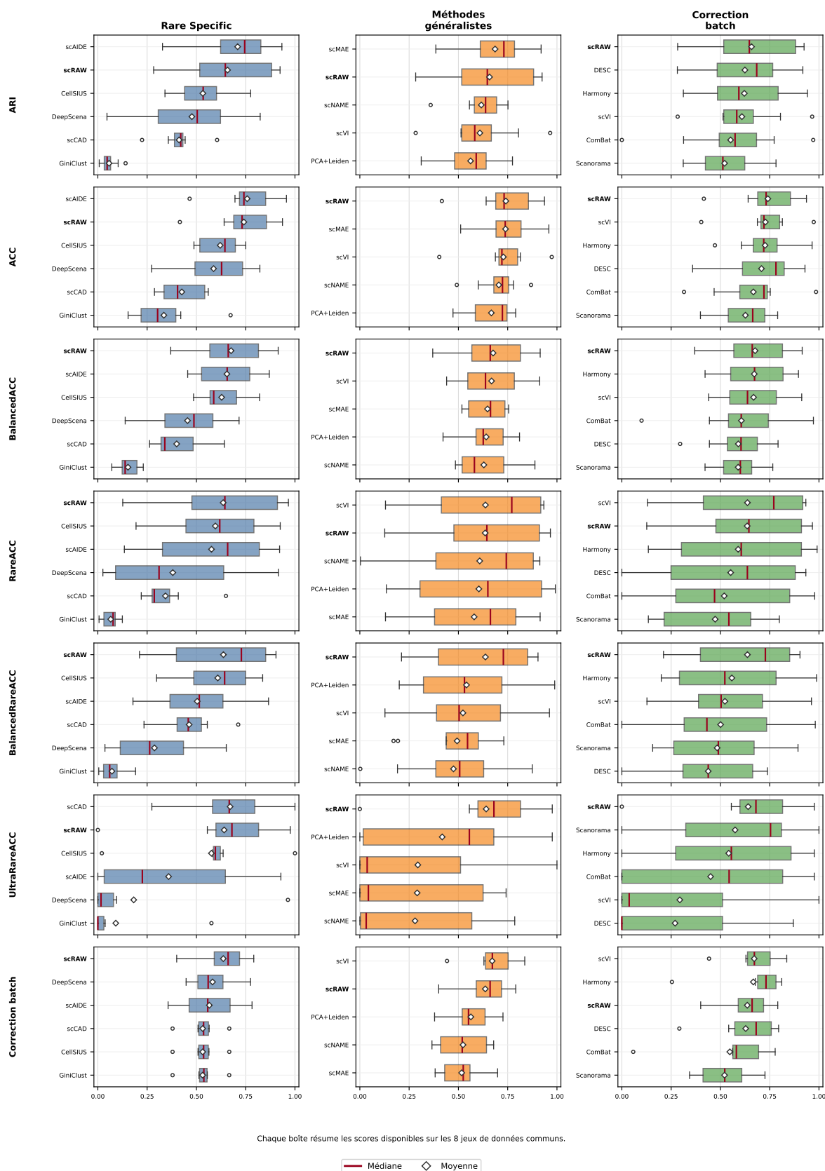
FIGURE 10 – Résultats complets par famille sur les 8 jeux de données communs. Les boîtes résument la distribution des scores pour ces 8 jeux de données par méthode ; les jeux sans classe ultra-rare ne contribuent pas à l'UltraRareACC. scRAW est ajouté comme repère dans chaque famille.
