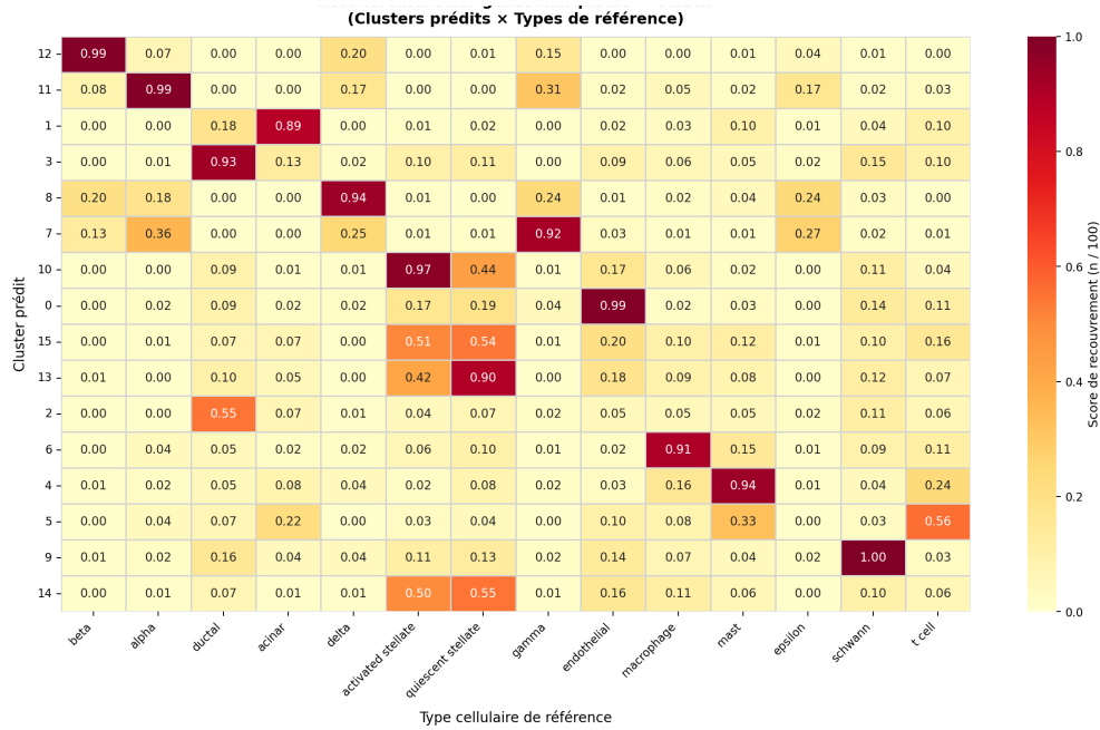
(b) Recouvrement des marqueurs. L'axe des ordonnées est ordonné par taille décroissante des clusters prédits, et l'axe des abscisses par taille décroissante des populations de référence (les cellules stellaires activées et quiescentes étant placées côte à côte pour faciliter la comparaison).
