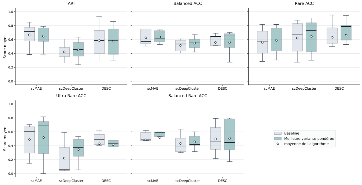
FIGURE 6 – Comparaison entre les algorithmes de base et leur meilleure variante avec loss pondérée scRAW. Les scores sont des moyennes sur les 5 jeux de données disponibles en Annexe E.
