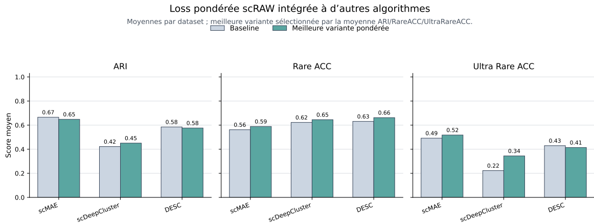
FIGURE 5 – Comparaison entre les algorithmes de base et leur meilleure variante avec loss pondérée scRAW. Les scores sont des moyennes par jeu de données.
