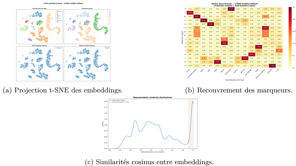
FIGURE 7 – Analyse biologique compacte de scRAW sur Baron Human Pancreas. Les panneaux combinent la structure latente, la concordance des marqueurs différentiels et la distribution des similarités de représentation afin d'évaluer la cohérence biologique du clustering sans dépasser une demi-page.
