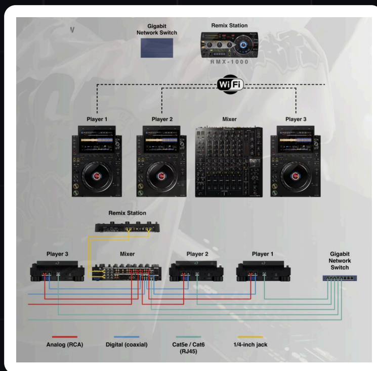
Esquema de ligações: três leitores, mixer, remix station e switch de rede. Analógico (RCA), digital coaxial, Cat5e/Cat6 (RJ45) e jack de 1/4.
