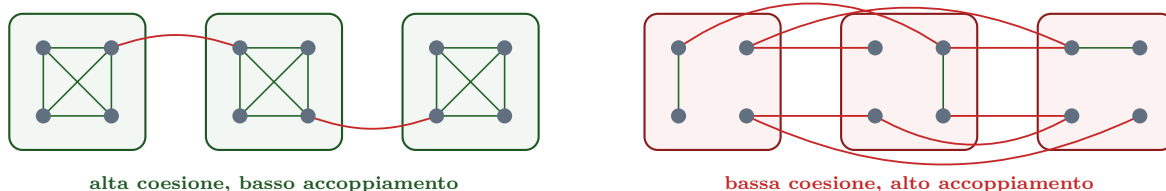
Figura 11.2: Gli stessi elementi raggruppati in due modi. In verde i legami interni ai moduli, in rosso quelli fra moduli. A sinistra ogni modulo è quasi autosufficiente; a destra quasi ogni legame attraversa i confini.
