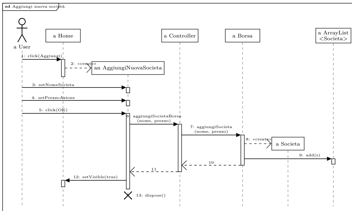
Figura 8.1: Il diagramma di sequenza di «Aggiungi nuova società», ricavato dal codice.
