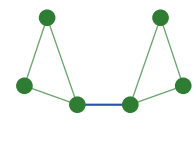
scomposti: 7 legami
