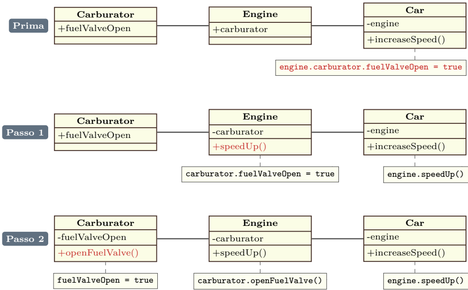
Figura 11.3: Eliminare il codice di navigazione. A ogni passo un oggetto smette di frugare nella struttura di un altro e gli chiede invece un servizio (in rosso i metodi aggiunti; nelle note il codice dei metodi).
