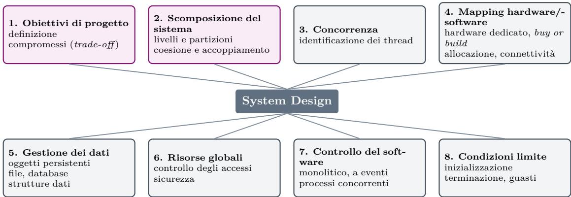
Figura 11.1: Gli otto aspetti del System Design. In questo capitolo: obiettivi di progetto e scomposizione.
