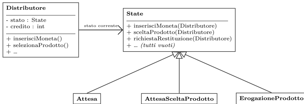
Figura 9.2: Il pattern State applicato al distributore: una sottoclasse di State per ogni stato del diagramma.
