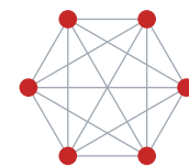
insieme: 15 legami
