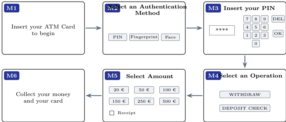
Figura 6.2: I mock-up M1–M6 del prelievo al bancomat, nell’ordine del main scenario.
