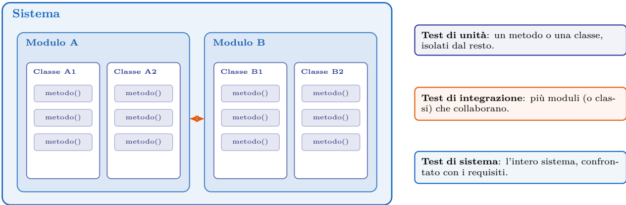
Figura 3.5: I livelli del test funzionale, dal più piccolo al più grande.
