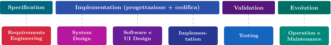
Figura 3.2: Corrispondenza tra le quattro attività fondamentali e le sei fasi del modello a cascata.
