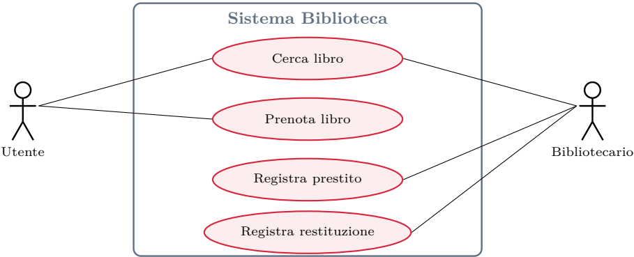
Esempio 3.1 — Un diagramma dei casi d'uso per la biblioteca
