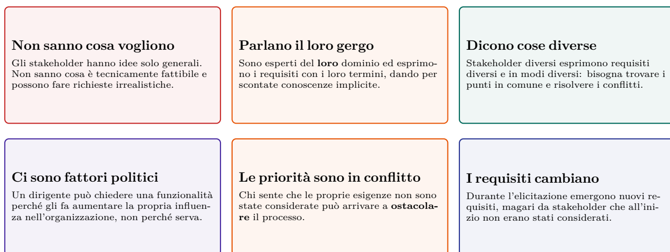
Figura 5.7: Le sei principali difficoltà dell'elicitazione dei requisiti.
