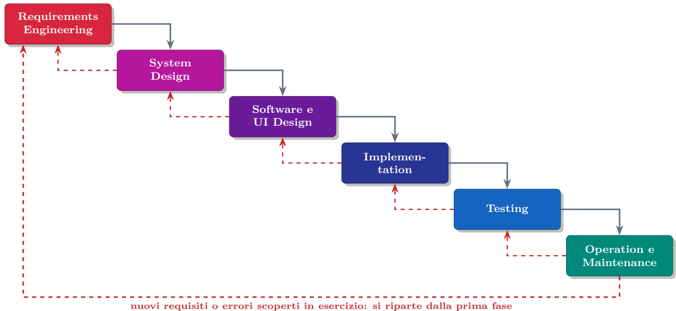
Figura 3.6: Nella realtà ogni fase può rimandare a quelle precedenti (freccie tratteggiate).
