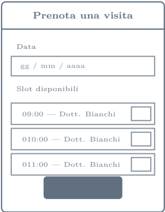
Figura 5.9: Un wireframe non deve essere bello: deve far capire struttura e flusso.
