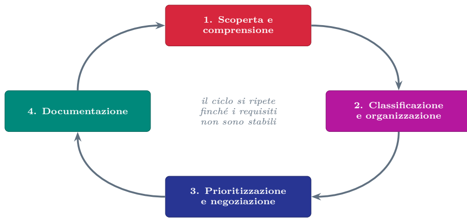
Figura 5.8: Il ciclo di elicitazione e analisi dei requisiti.
