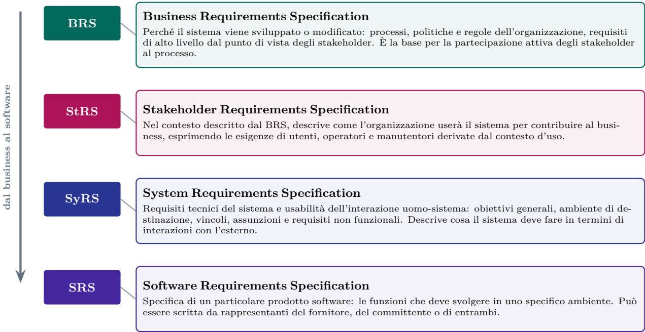
Figura 5.11: I quattro documenti previsti dallo standard ISO/IEC/IEEE 29148:2018.
