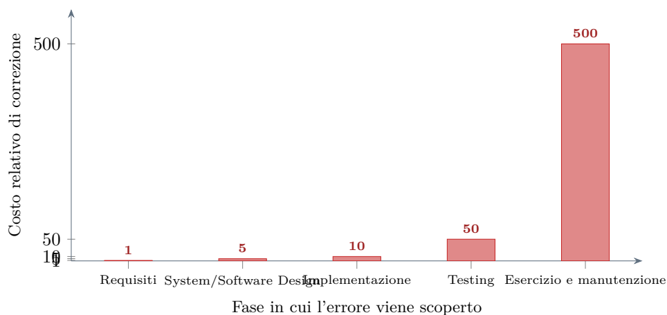
Figura 3.7: Costo relativo per correggere un errore, in funzione della fase in cui viene scoperto (B. W. Boehm, Software Engineering Economics ).
