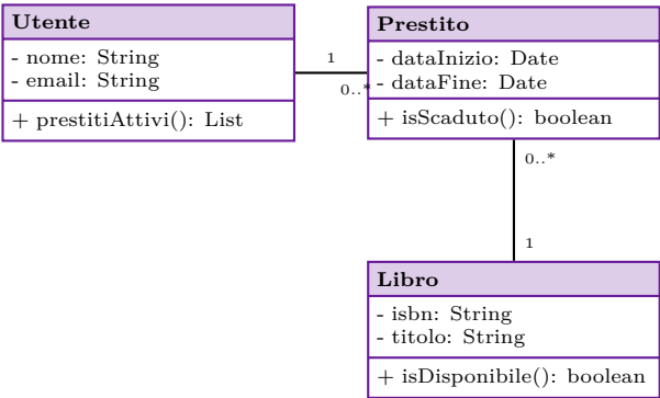
(a) Diagramma delle classi UML
