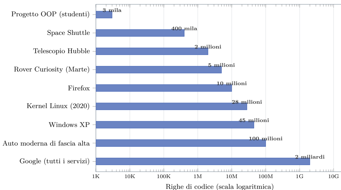
Figura 1.2: Ordini di grandezza del software reale (stime diffuse pubblicamente, arrotondate).
