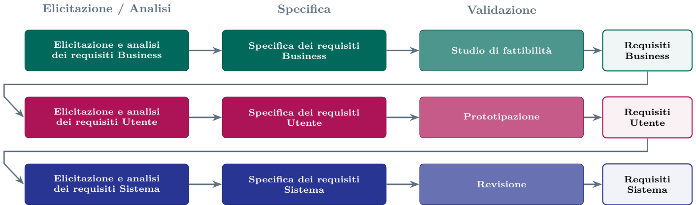
Figura 5.5: Il processo iterativo: ogni livello di requisiti attraversa le tre attività e alimenta il livello successivo.
