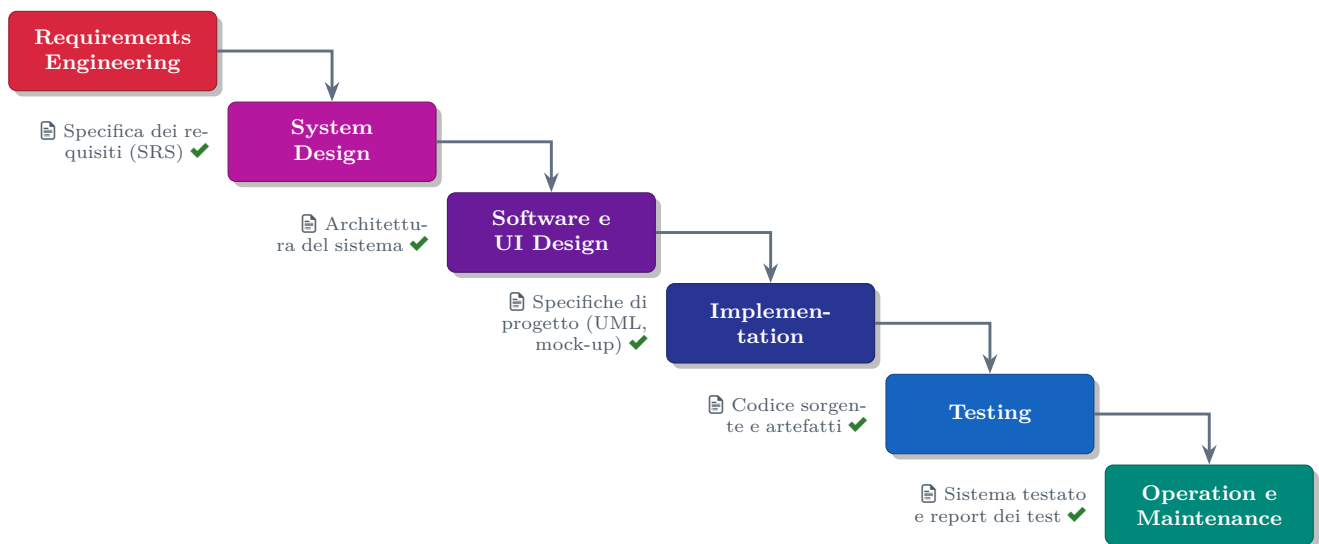
Figura 3.1: Il modello a cascata. A sinistra di ogni fase, il documento (approvato) prodotto dalla fase precedente.
