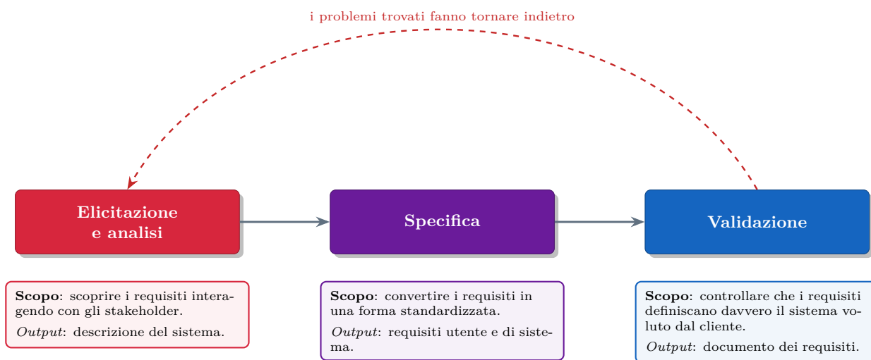
Figura 5.4: Le tre attività del processo di Requirements Engineering.
