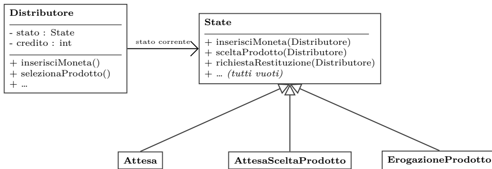
Figura 7.2: Il pattern State applicato al distributore: una sottoclasse di State per ogni stato del diagramma.
