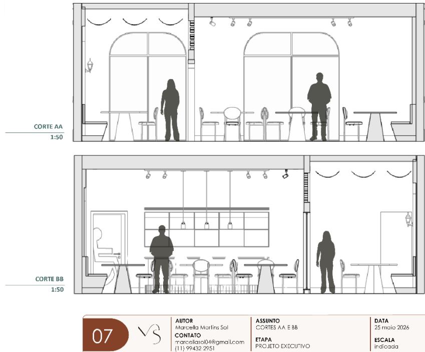
Figura 12: Corte AA e Corte BB
