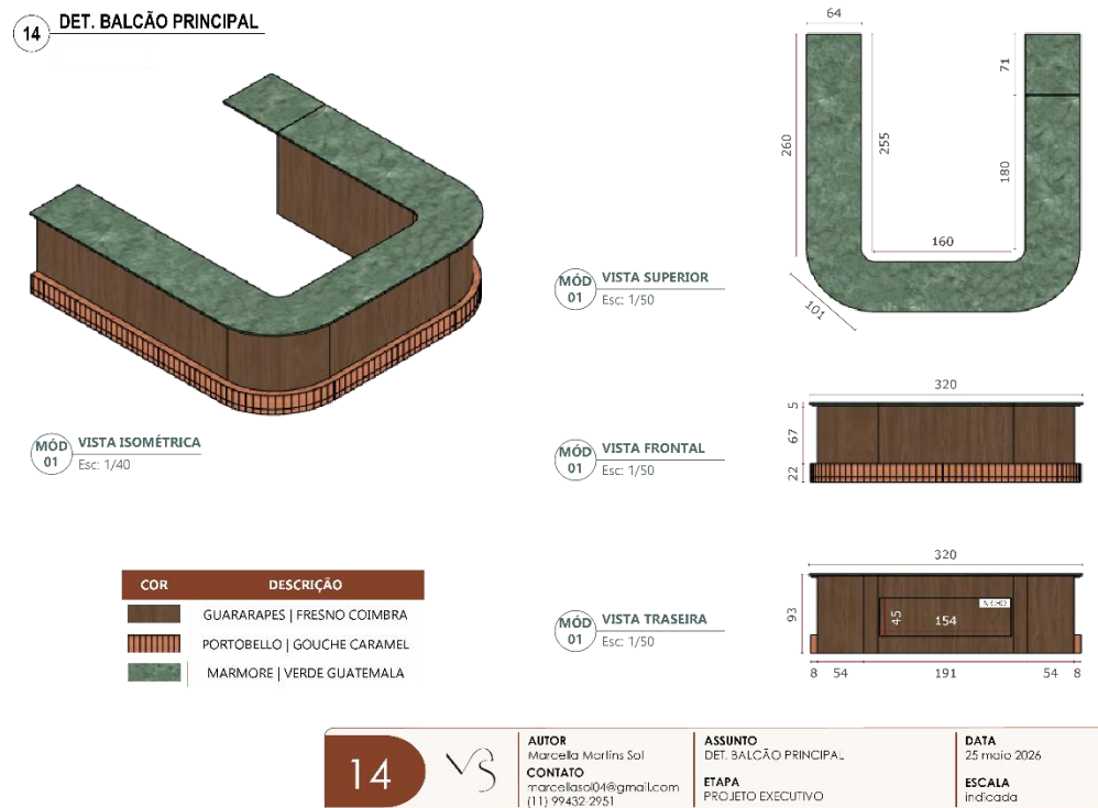
Figura 21: Detalhamento do Balcão em U
