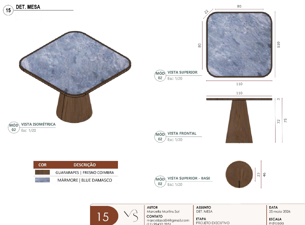
Figura 22: Detalhamento de Mesa
