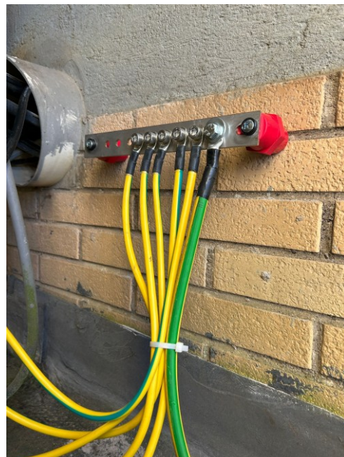
Messe a terra esterne
