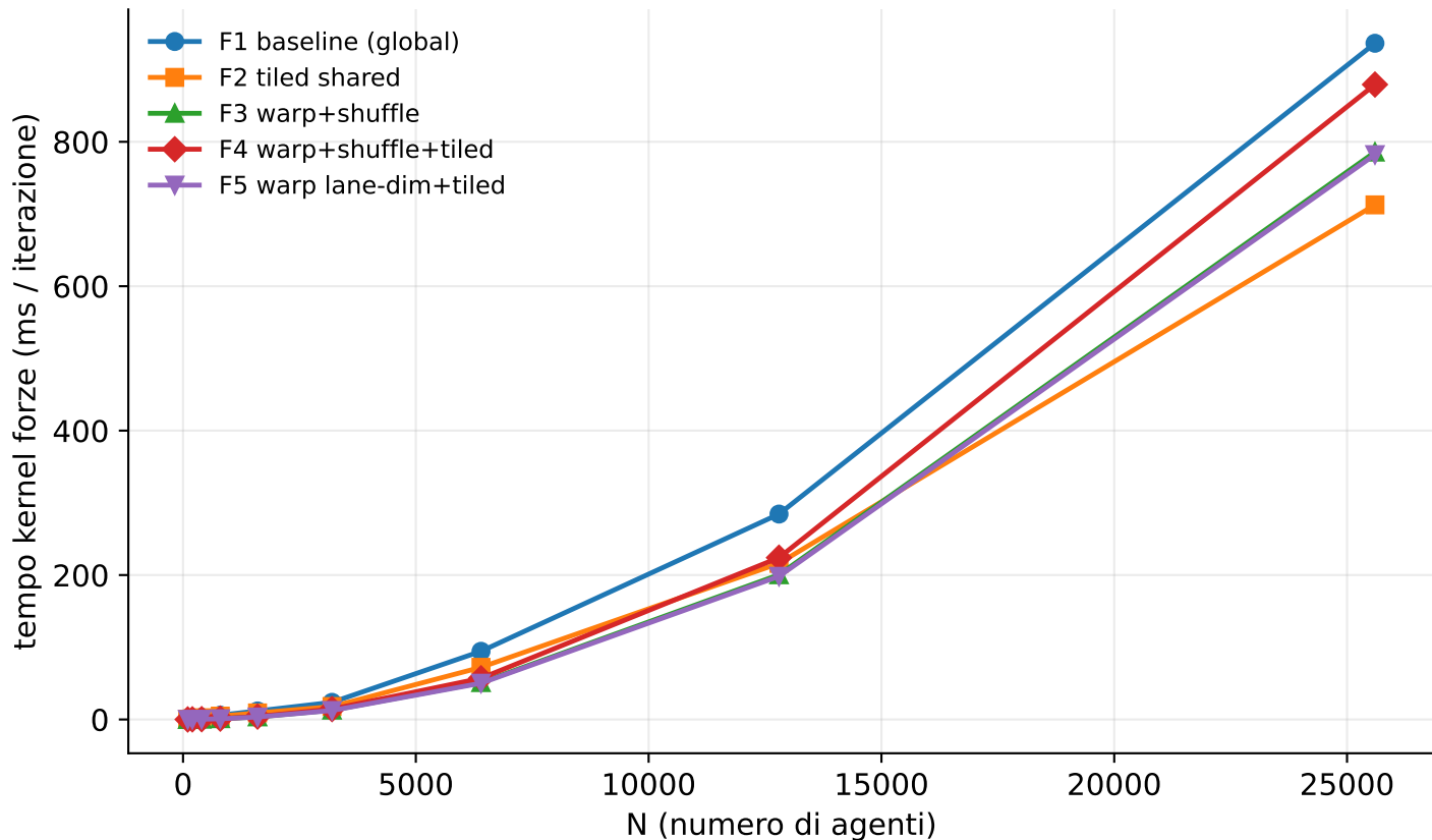
Kernel force: 5 versioni CUDA al variare di N — K=64 NC=512 DEG=3
