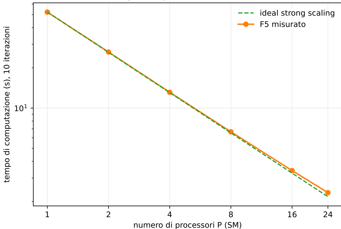
Strong scaling — F5, N = 12800 fisso
