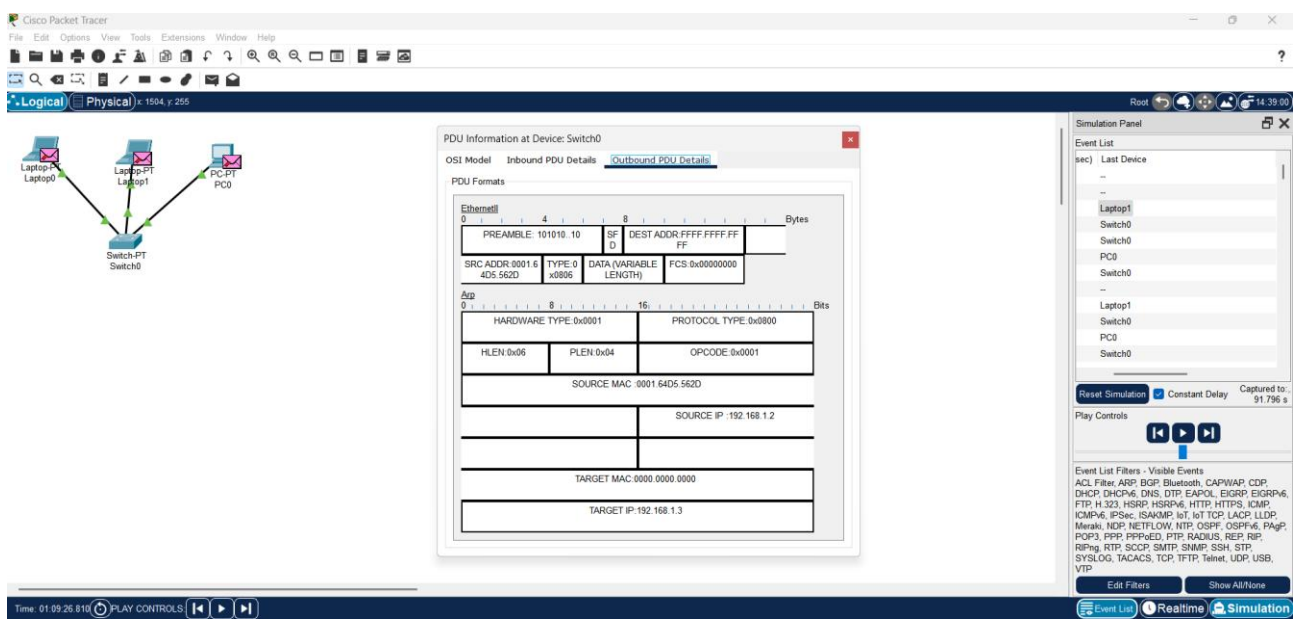
Figura 3 Qui invece vediamo come è composto il pacchetto, qual è il suo Header e quale il suo Payload, contenuto, da quanti bit composto
