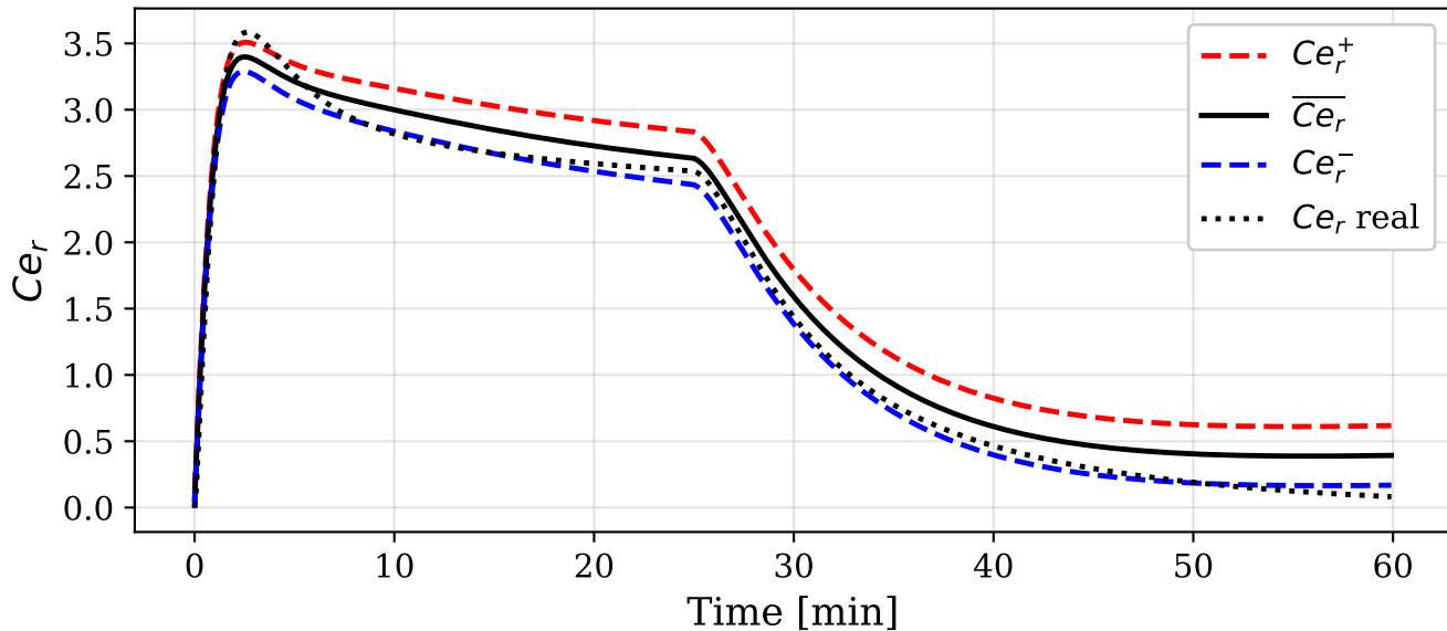
Concentración de remifentanilo en sitio de efecto
