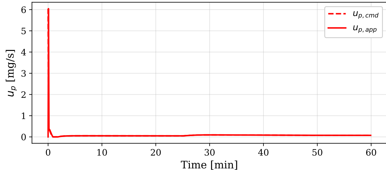
Propofol comandado vs aplicado
