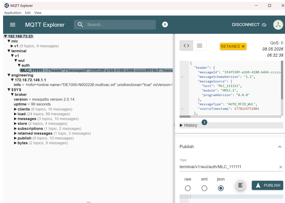
Abbildung 3.2: MQTT Explorer
