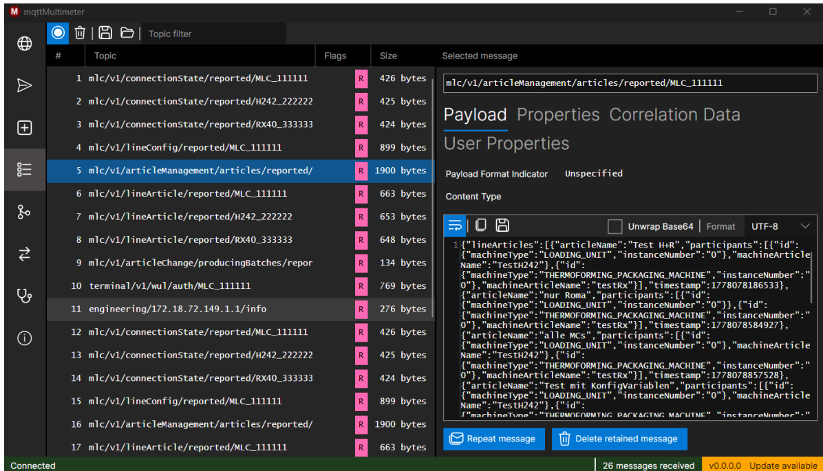
Abbildung 3.4: Nachrichtenverlauf im MQTTMultimeter
