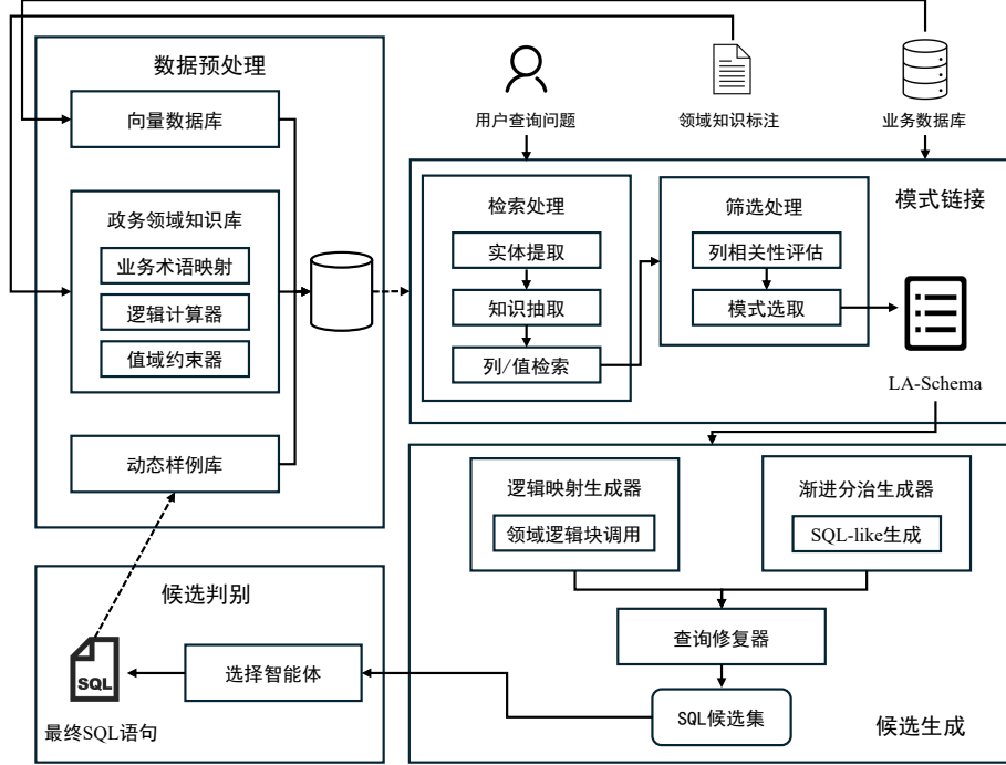
图 4-1 逻辑增强与异构协同的 Text-to-SQL 框架图
