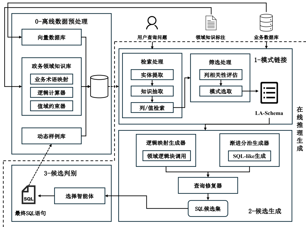
图 3-1 逻辑增强与异构协同的 Text-to-SQL 框架图
