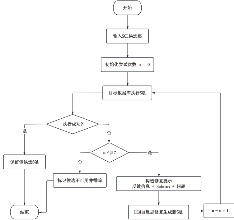
图 3-3 查询修复流程图
