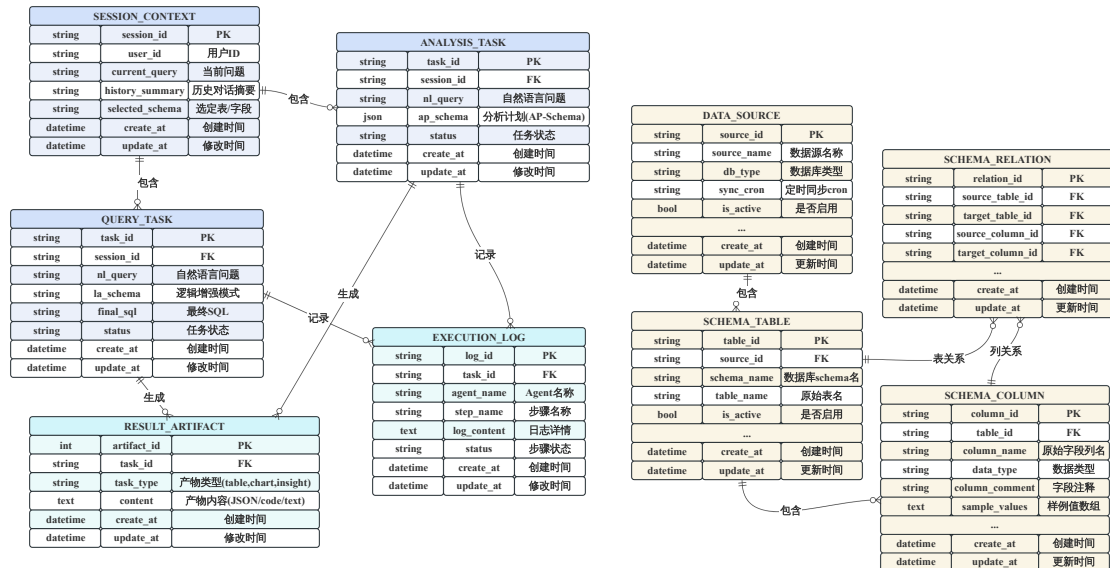
图 5-5 系统元数据库 ER 图
