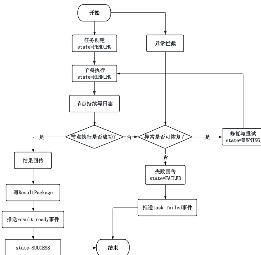
图 5-3 异常处理与结果回传实现图
