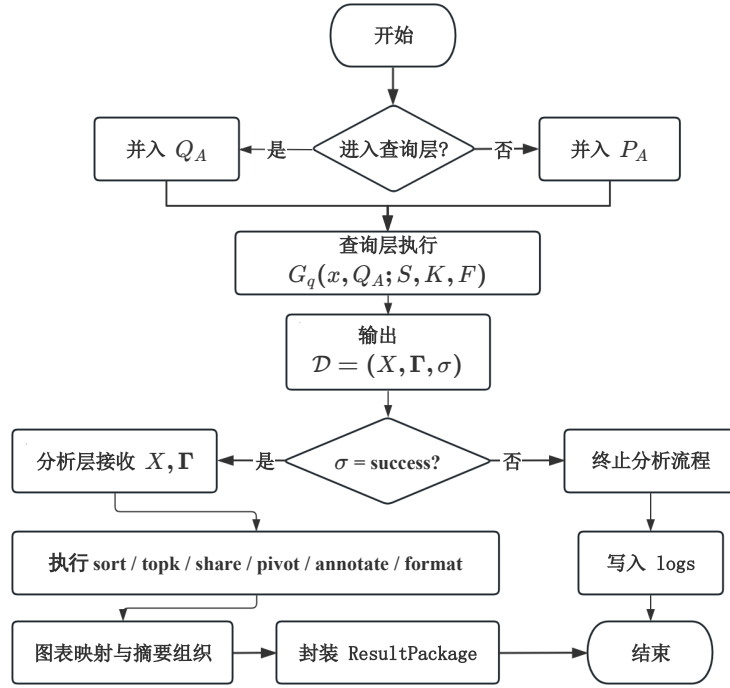
图 4-4 层间衔接流程图
