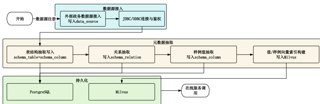
图 5-4 业务数据源接入与元数据抽取实现图
