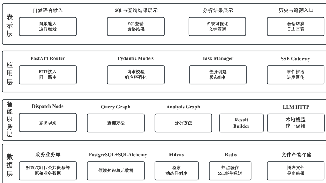
图 5-1 系统总体分层架构图
