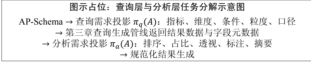
图 4-2 查询层与分析层任务分解示意图
