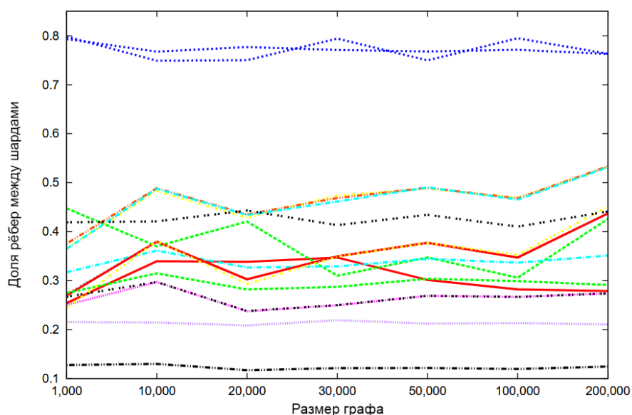
Рис. 5: Визуализация доли рёбер между шардами для 4 шардов с порядком BFS. Нижняя линия - METIS, предпоследняя линия - Лин. Дет. жадная [7]
