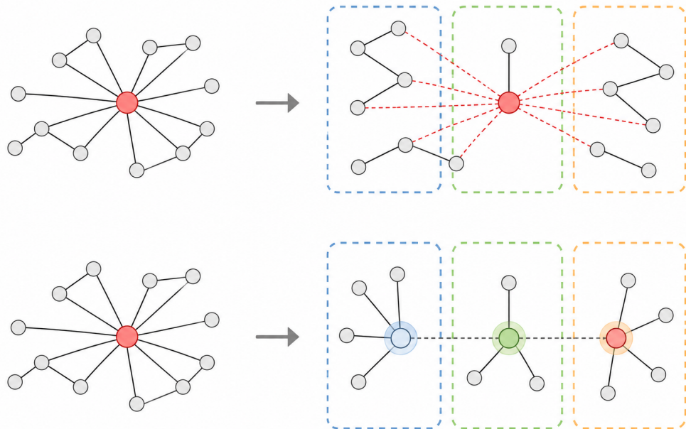
Рис. 5: Вершина-хаб. Нерациональное хранение с множеством межшардовых переходов (сверху), уменьшение переходов через дублирование (снизу)
