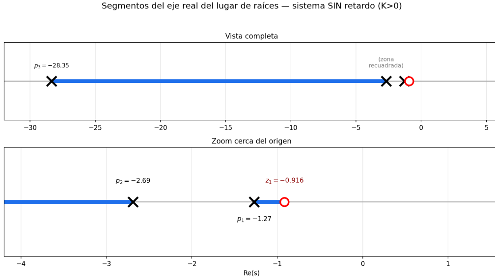
Figura 9: Segmentos entre polos y ceros para el caso sin retardo.
