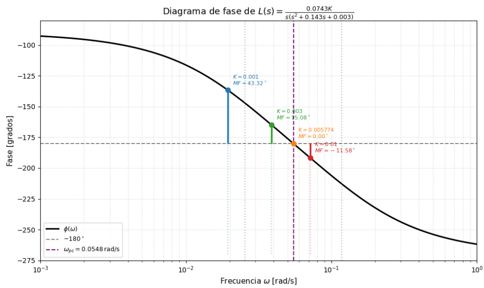
Figura 9: Diagrama de fase de L(s) y márgenes de fase correspondientes a las ganancias seleccionadas. La fase no depende de K para K > 0 .
