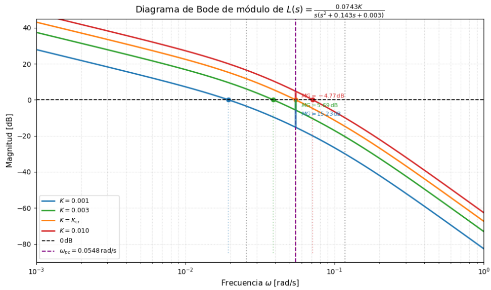
Figura 8: Diagrama de Bode de módulo de L(s) para distintas ganancias. Los márgenes de ganancia se determinan en \omega_{pc} \approx 0,05477226 rad/s.
