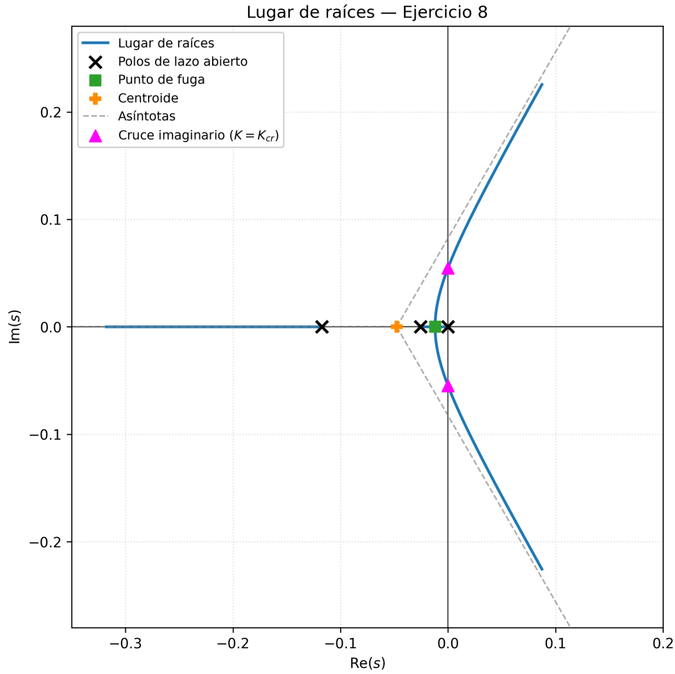
Figura 15: Lugar de raíces del sistema compensado de la incubadora neonatal para K \geq 0 . Se muestran los polos de lazo abierto, el punto de fuga s_f = -0,012 , el centroide, las asíntotas y el cruce del eje imaginario para K = K_{cr} .
