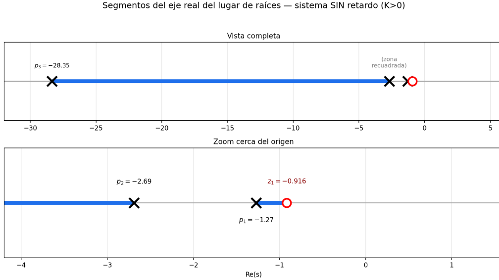
Figura 13: Segmentos entre polos y ceros para el caso sin retardo.
