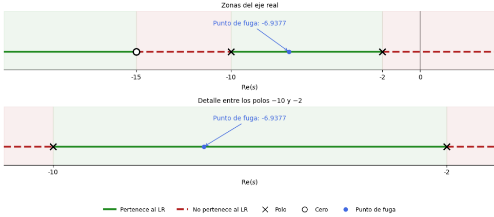
Figura 3: Zonas del eje real pertenecientes al lugar de raíces para el sistema con cero adicional en s = -15 .
