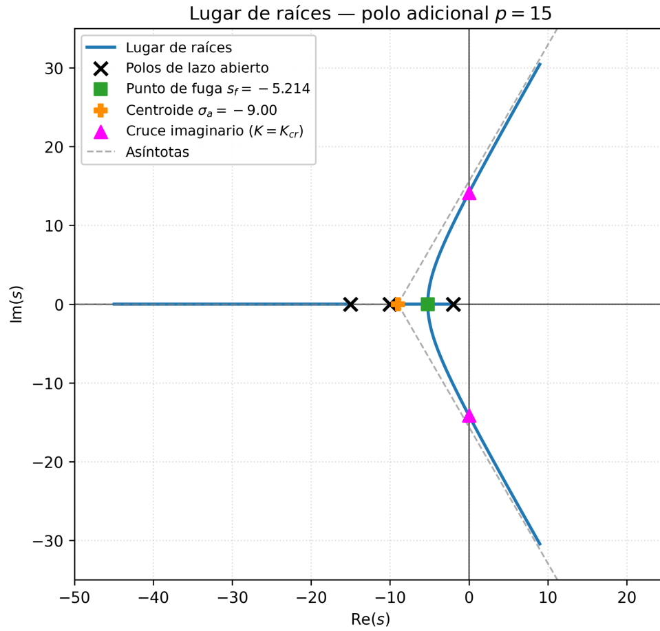
Figura 8: Lugar de raíces completo para el sistema con polo adicional en s = -15 . Se muestran los polos de lazo abierto, el punto de fuga s_f \approx -5,2141 , el centroide, las asíntotas y el cruce del eje imaginario en s \approx \pm j 14,1421 .
