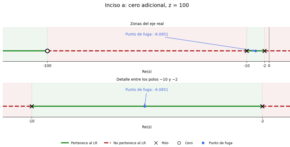
Figura 1: Zonas del eje real pertenecientes al lugar de raíces para el sistema con cero adicional en s = -100 .
