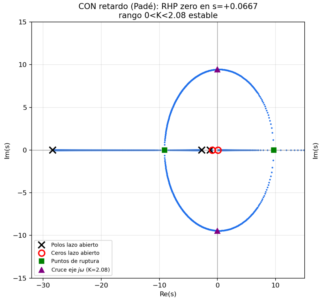
Figura 12: Gráfico del lugar de raíces, en el caso del sistema con retardo.
