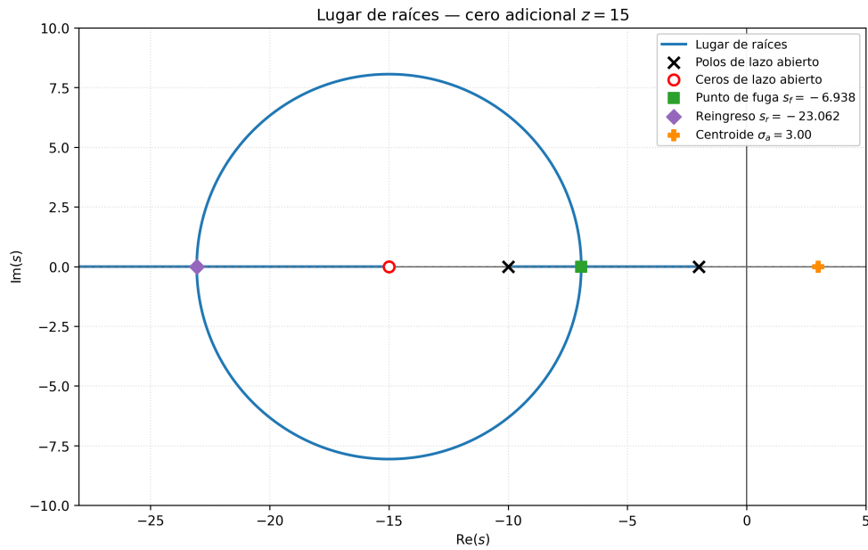
Figura 4: Lugar de raíces completo para el sistema con cero adicional en s = -15 . Las ramas parten de los polos -10 y -2 , se encuentran en s_f \approx -6,9377 , forman un par complejo conjugado y vuelven al eje real en s_r \approx -23,0623 . Una rama termina en el cero s = -15 y la otra se dirige hacia -\infty .
