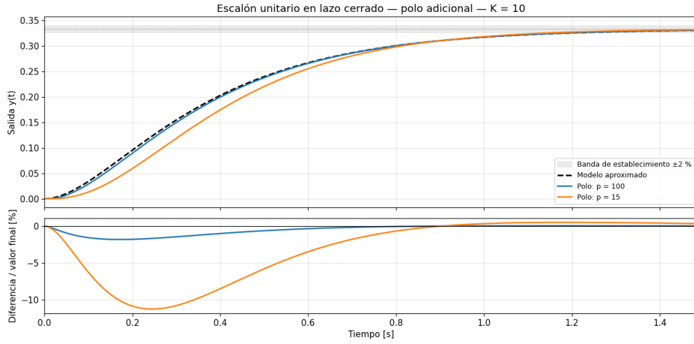
Figura 10: Respuesta al escalón unitario en lazo cerrado con polo adicional para p = 100 y p = 15 , comparada con el modelo aproximado, utilizando K = 10 . El panel inferior muestra la diferencia normalizada por el valor final común.
