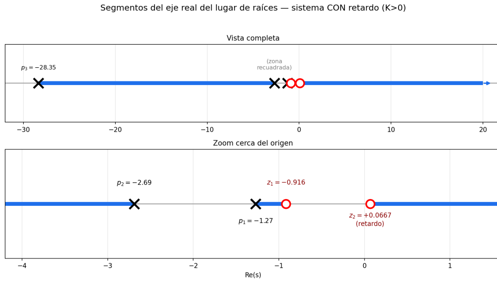
Figura 11: Segmentos entre polos y ceros para el caso con retardo.
