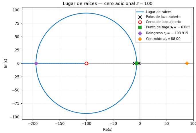
Figura 2: Lugar de raíces completo para el sistema con cero adicional en s = -100 . Las ramas parten de los polos -10 y -2 , se encuentran en s_f \approx -6,0851 , forman un par complejo conjugado y reingresan al eje real en s_r \approx -193,9149 . Una rama termina en el cero s = -100 y la otra se dirige hacia -\infty .
