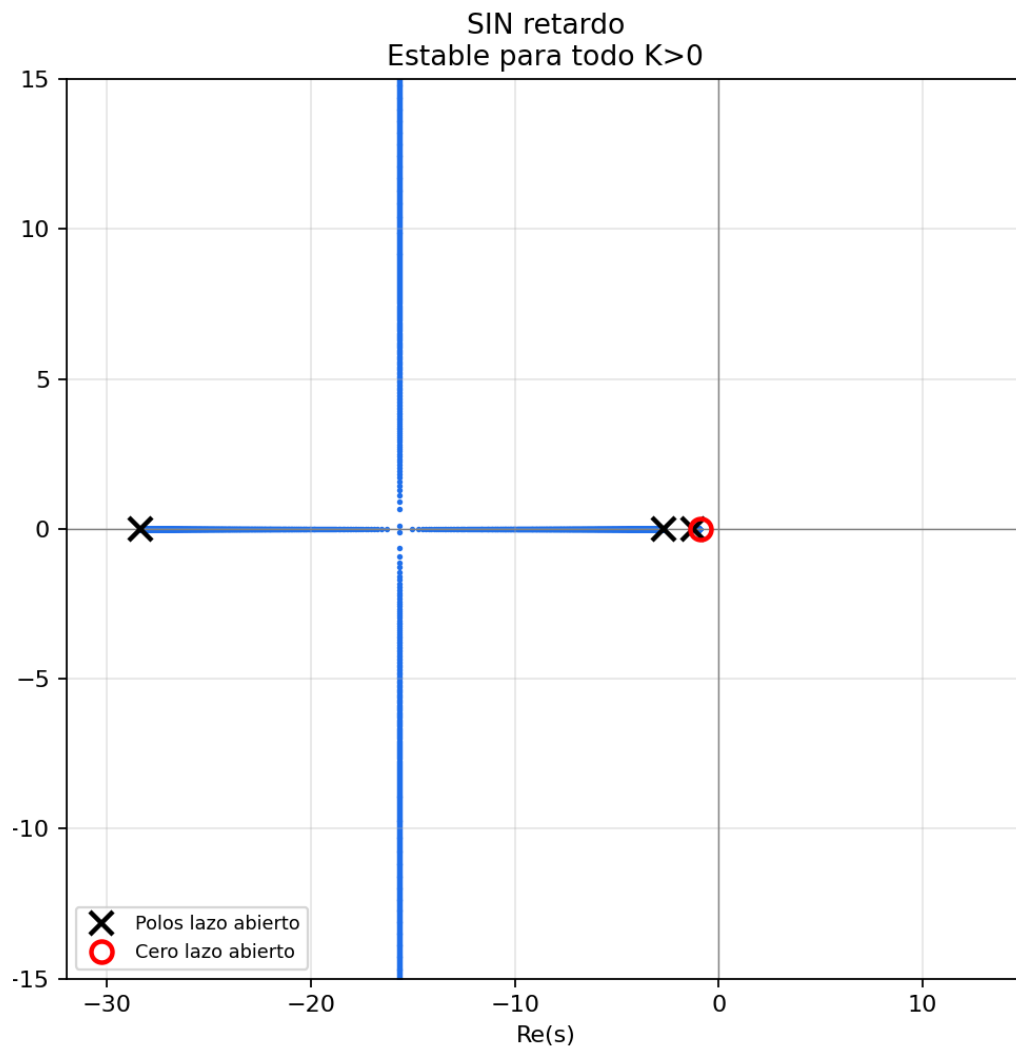
Figura 14: Gráfico del lugar de raíces, en el caso del sistema sin retardo.
