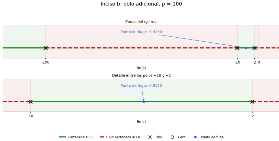
Figura 5: Zonas del eje real pertenecientes al lugar de raíces para el sistema con polo adicional en s = -100 .
