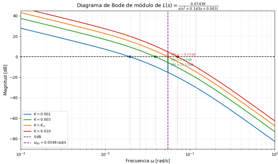
Figura 16: Diagrama de Bode de módulo de L(s) para distintas ganancias. Los márgenes de ganancia se determinan en \omega_{pc} \approx 0,05477226 \text{ rad/s} .
