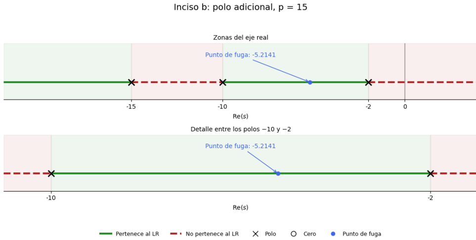
Figura 7: Zonas del eje real pertenecientes al lugar de raíces para el sistema con polo adicional en s = -15 .
