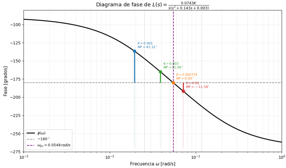
Figura 17: Diagrama de fase de L(s) y márgenes de fase correspondientes a las ganancias seleccionadas. La fase no depende de K para K > 0 .
