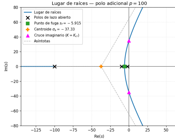
Figura 6: Lugar de raíces completo para el sistema con polo adicional en s = -100 . Se muestran los polos de lazo abierto, el punto de fuga s_f \approx -5,9150 , el centroide, las asíntotas y el cruce del eje imaginario en s \approx \pm j 34,9285 .
