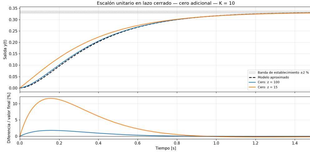
Figura 9: Respuesta al escalón unitario en lazo cerrado con cero adicional para z = 100 y z = 15 , comparada con el modelo aproximado, utilizando K = 10 . El panel inferior muestra la diferencia normalizada por el valor final común.
