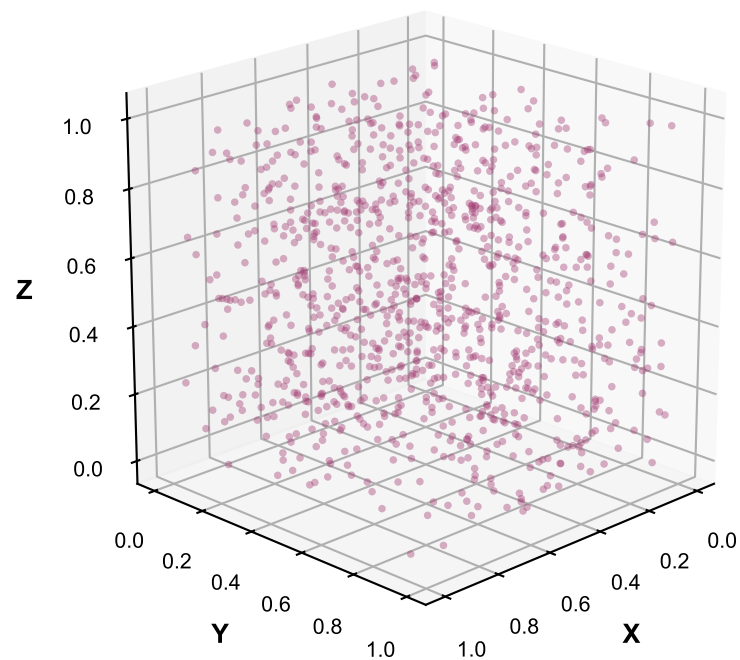
(D) "Deck of Cards": H > 0 (6 planes)
