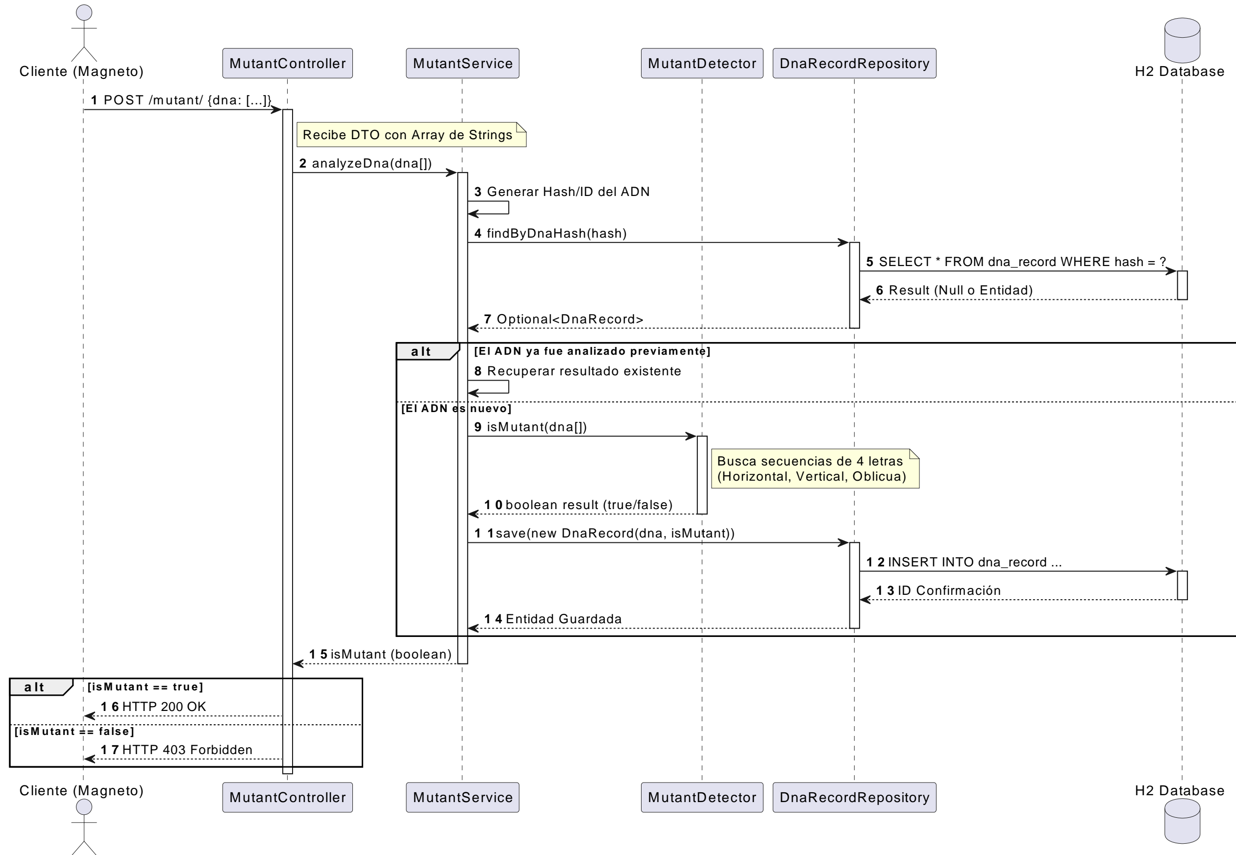
Diagrama de Secuencia: Detección de Mutantes (POST /mutant/)
