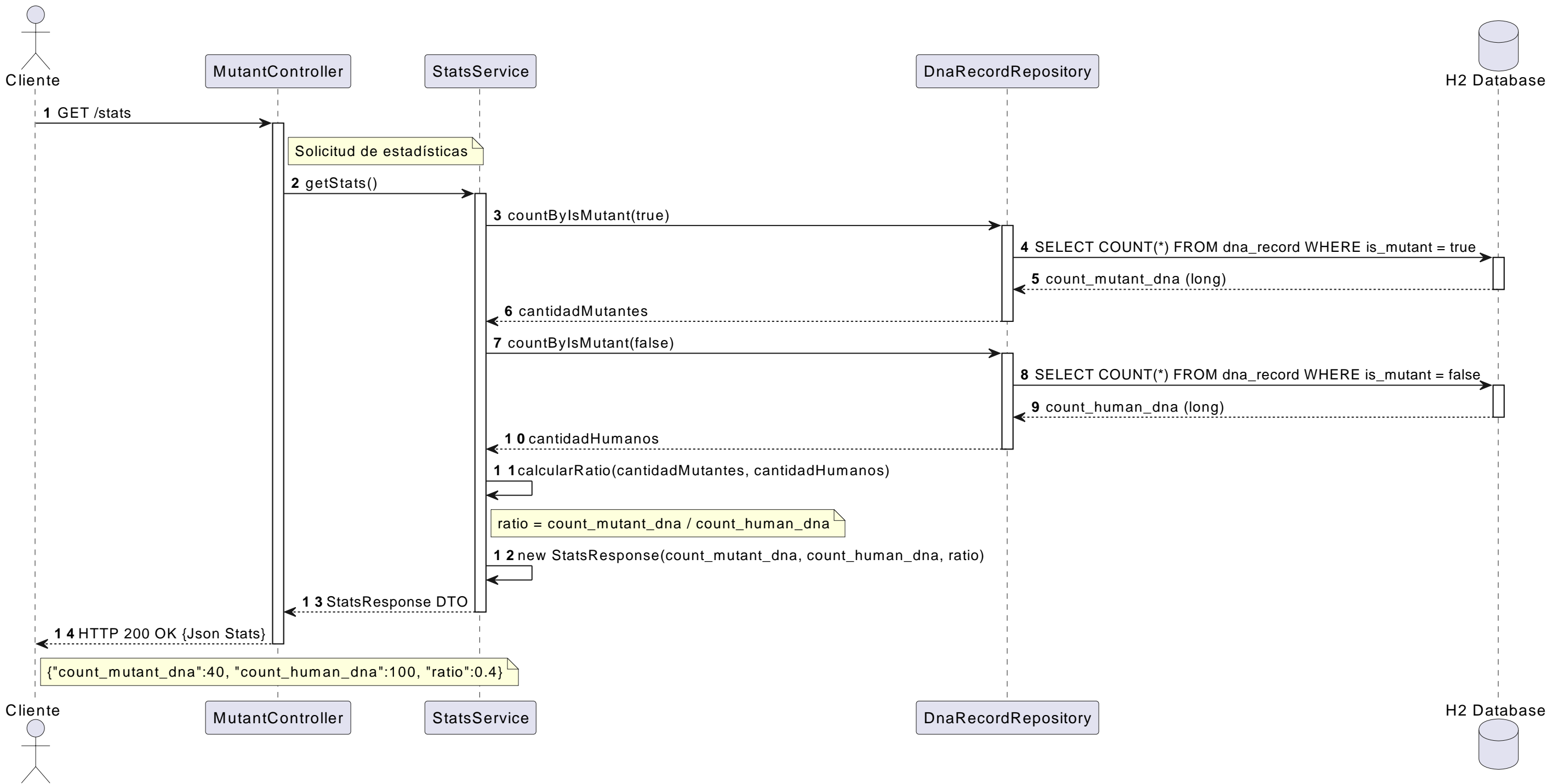
Diagrama de Secuencia: Estadísticas (GET /stats)
