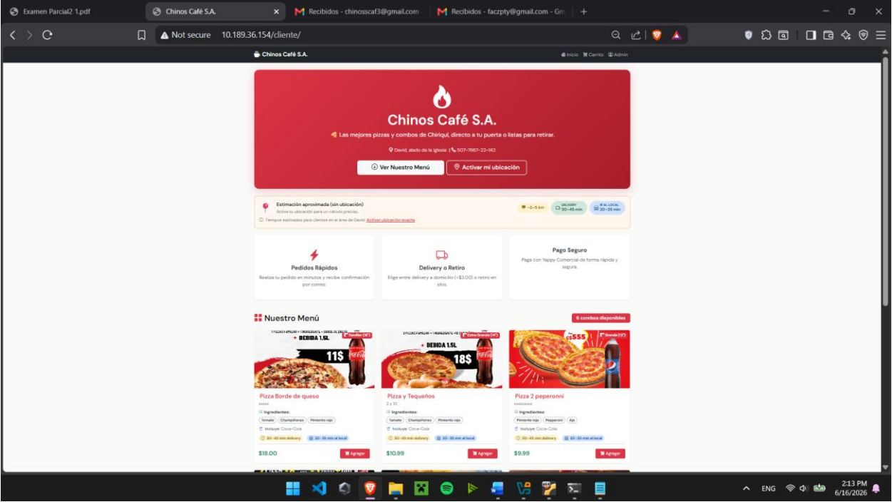
Servidor web
