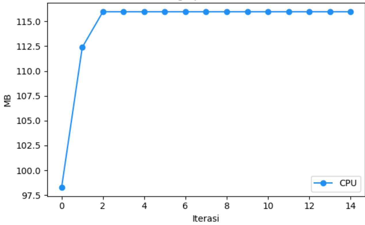
RAM Usage per Iterasi (CPU)
