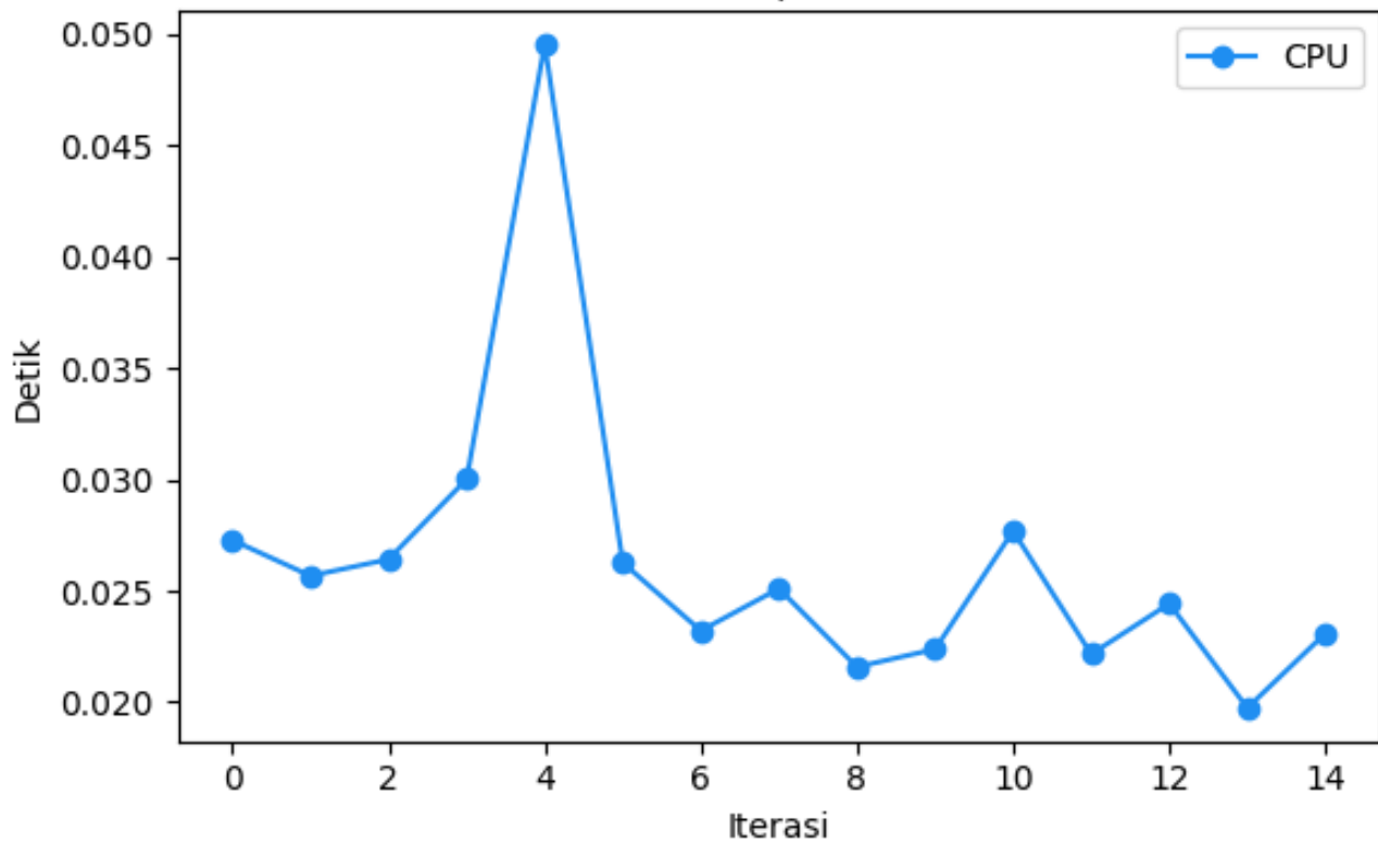
Waktu Inferensi per Iterasi (CPU)
