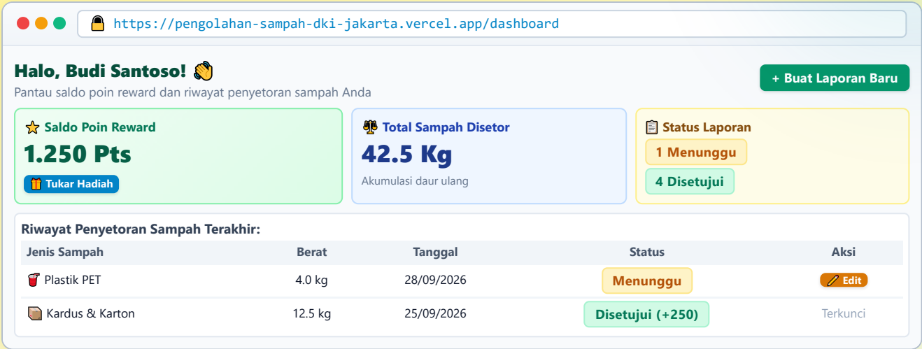
Gambar 8.1 Tampilan Layar Dashboard Utama Akun Warga SampahKu
