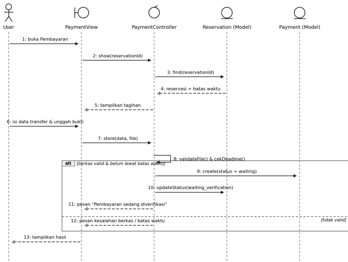
Gambar 3.21 Sequence diagram #7 Melakukan Pembayaran
