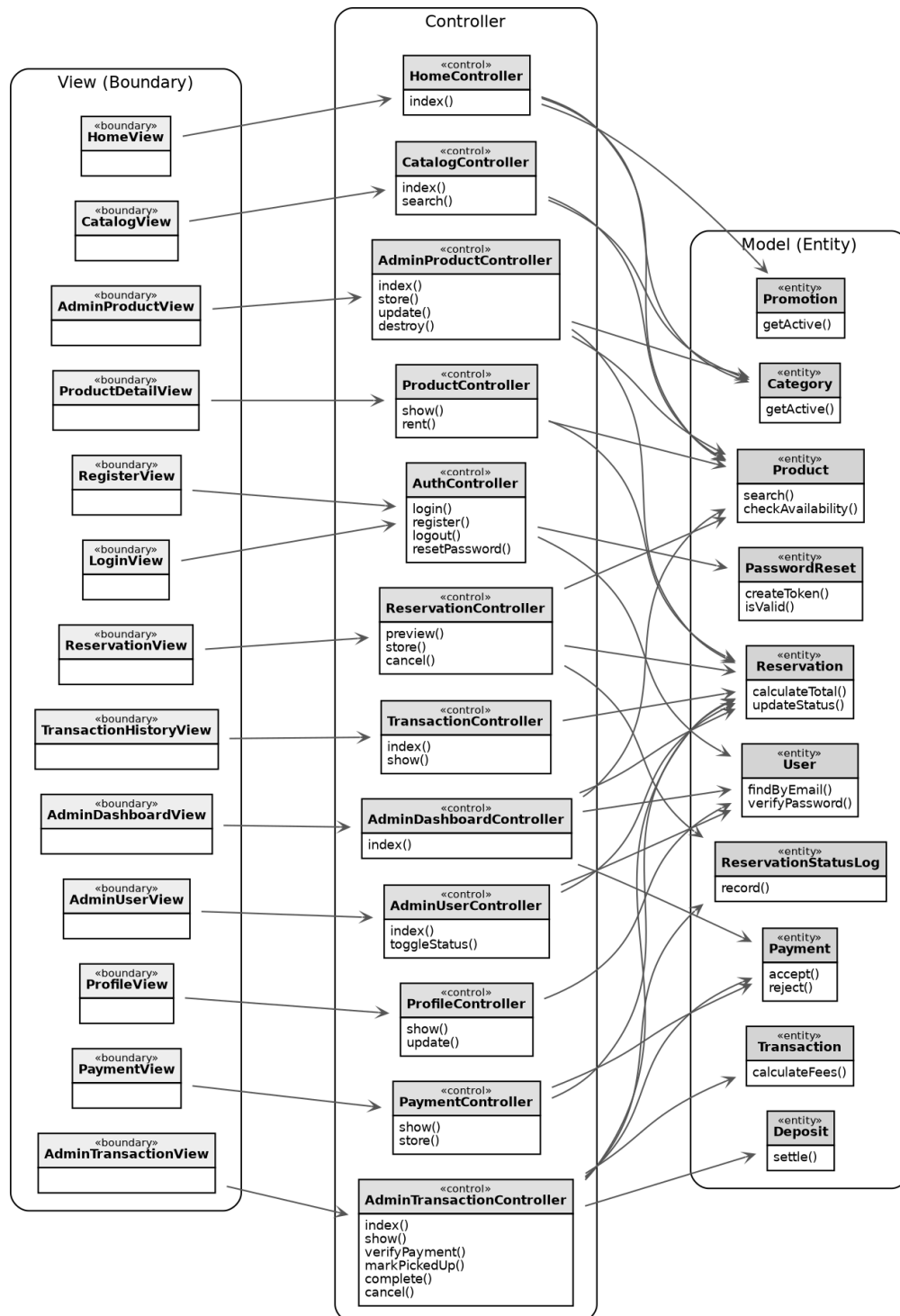
Gambar 3.41 Diagram kelas keseluruhan (MVC)
