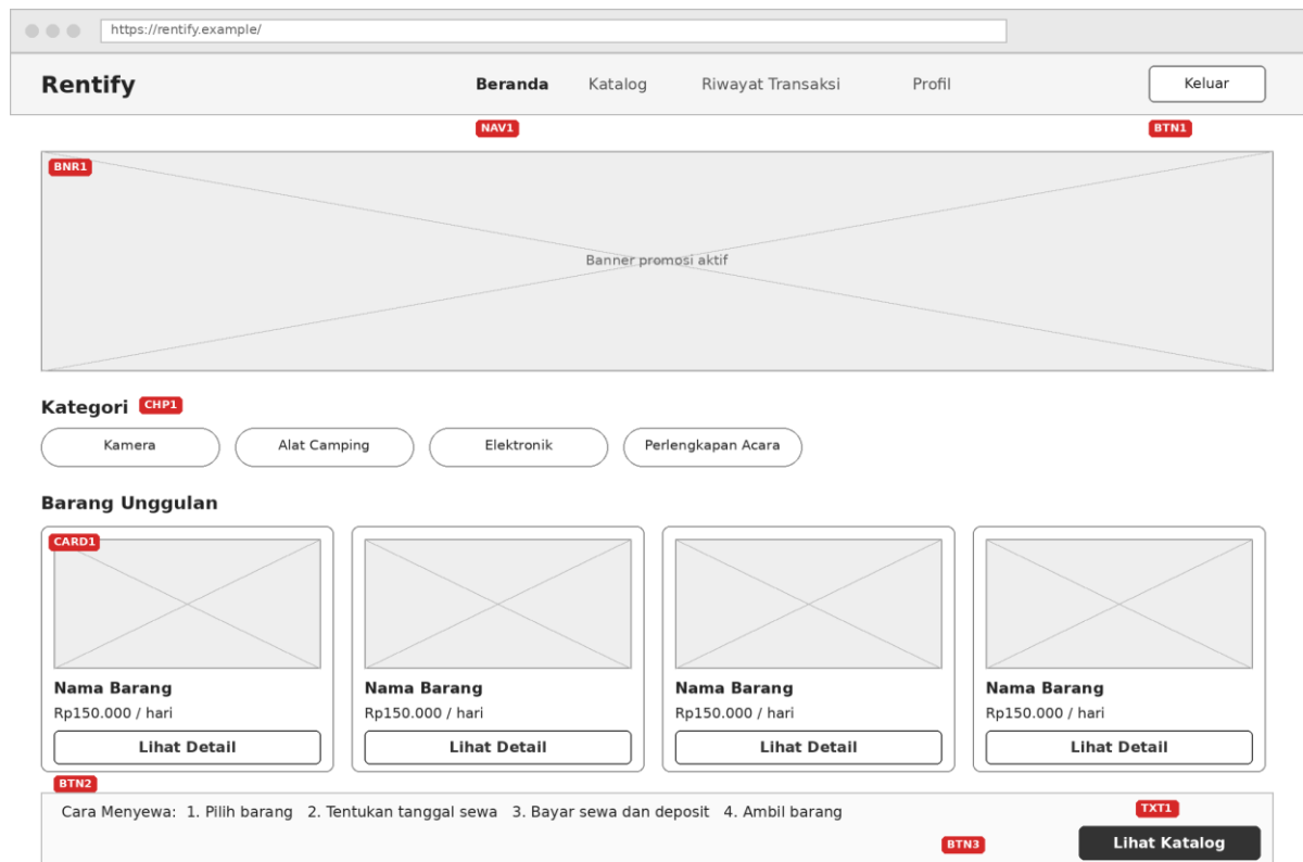
Gambar 3.8 Rancangan antarmuka P01 Beranda
