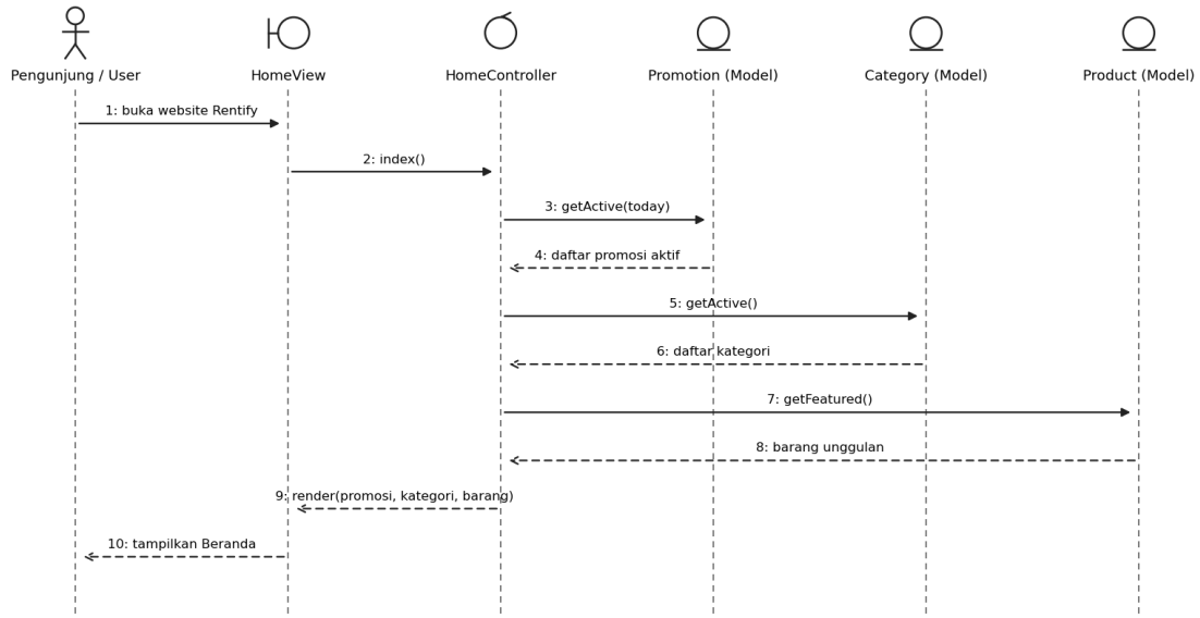
Gambar 3.9 Sequence diagram #3 Melihat Beranda
