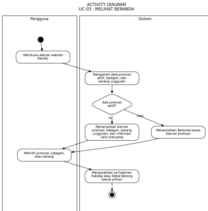
Gambar 3.10 Activity diagram #3 Melihat Beranda
