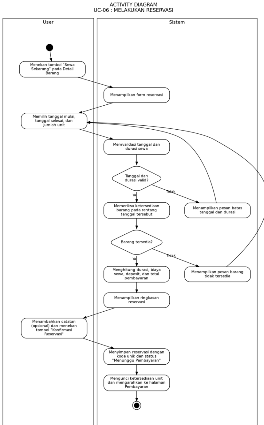
Gambar 3.19 Activity diagram #6 Melakukan Reservasi
