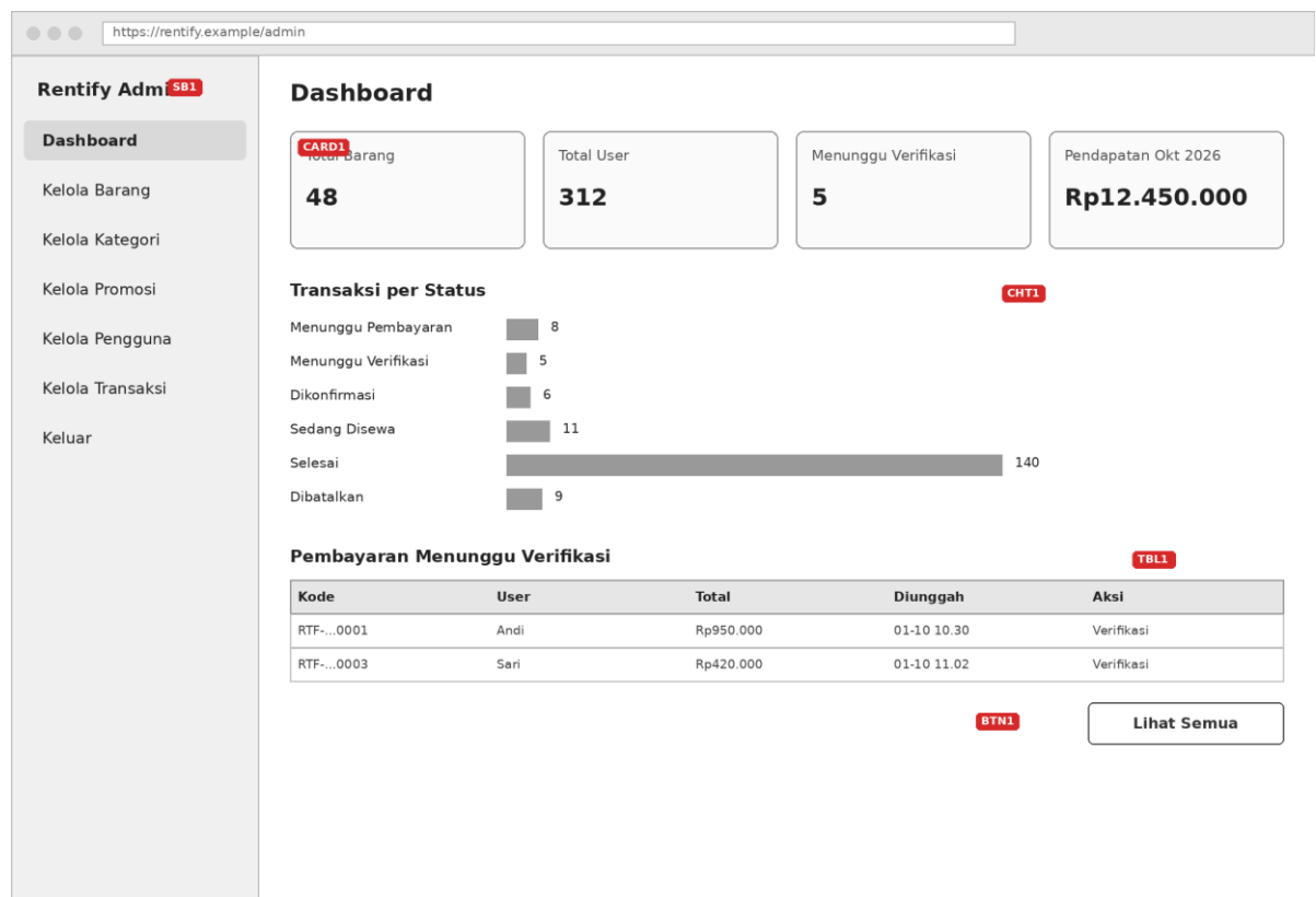
Gambar 3.29 Rancangan antarmuka P10 Admin Dashboard
