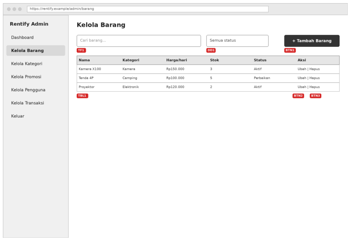
Gambar 3.30 Rancangan antarmuka P11 Kelola Barang
