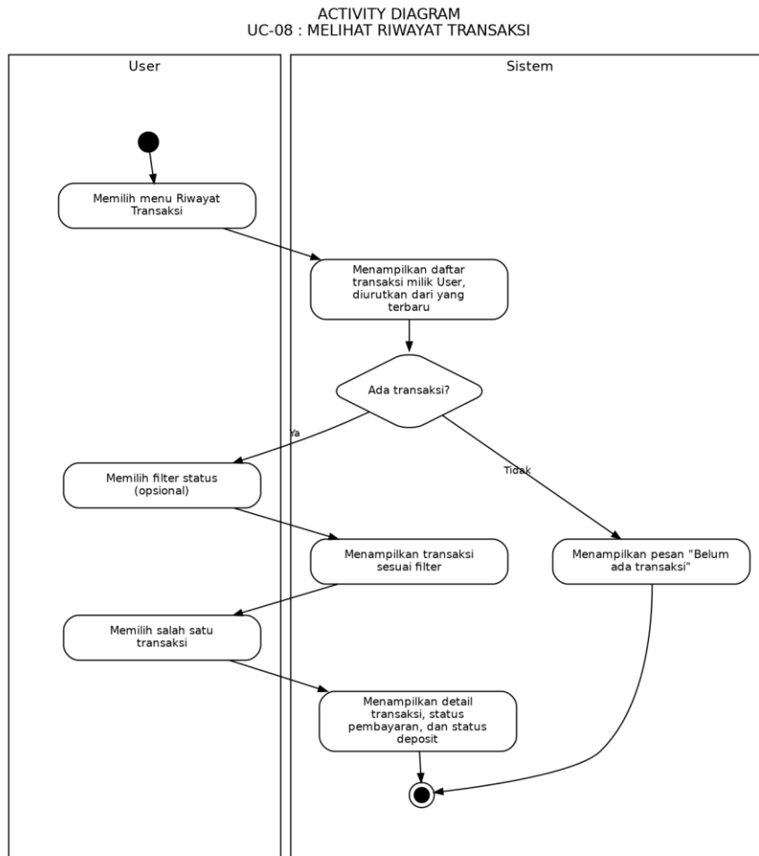
Gambar 3.25 Activity diagram #8 Melihat Riwayat Transaksi
