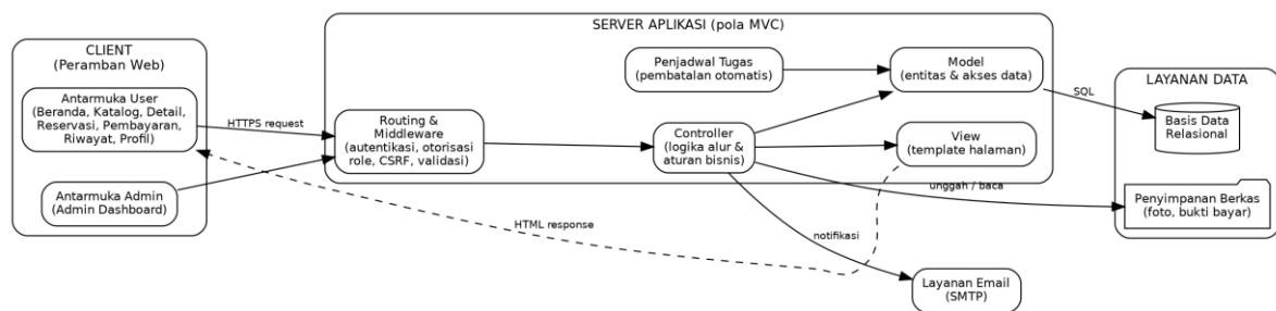
Gambar 2.1 Arsitektur sistem Rentify
