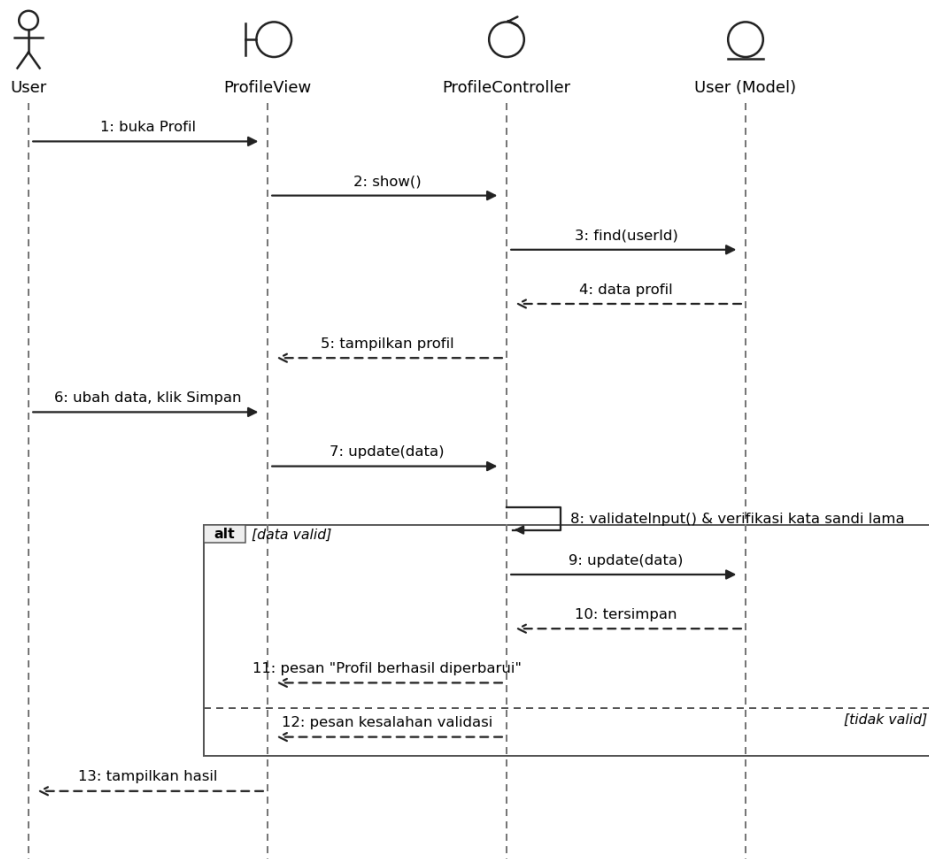
Gambar 3.27 Sequence diagram #9 Mengelola Profil
