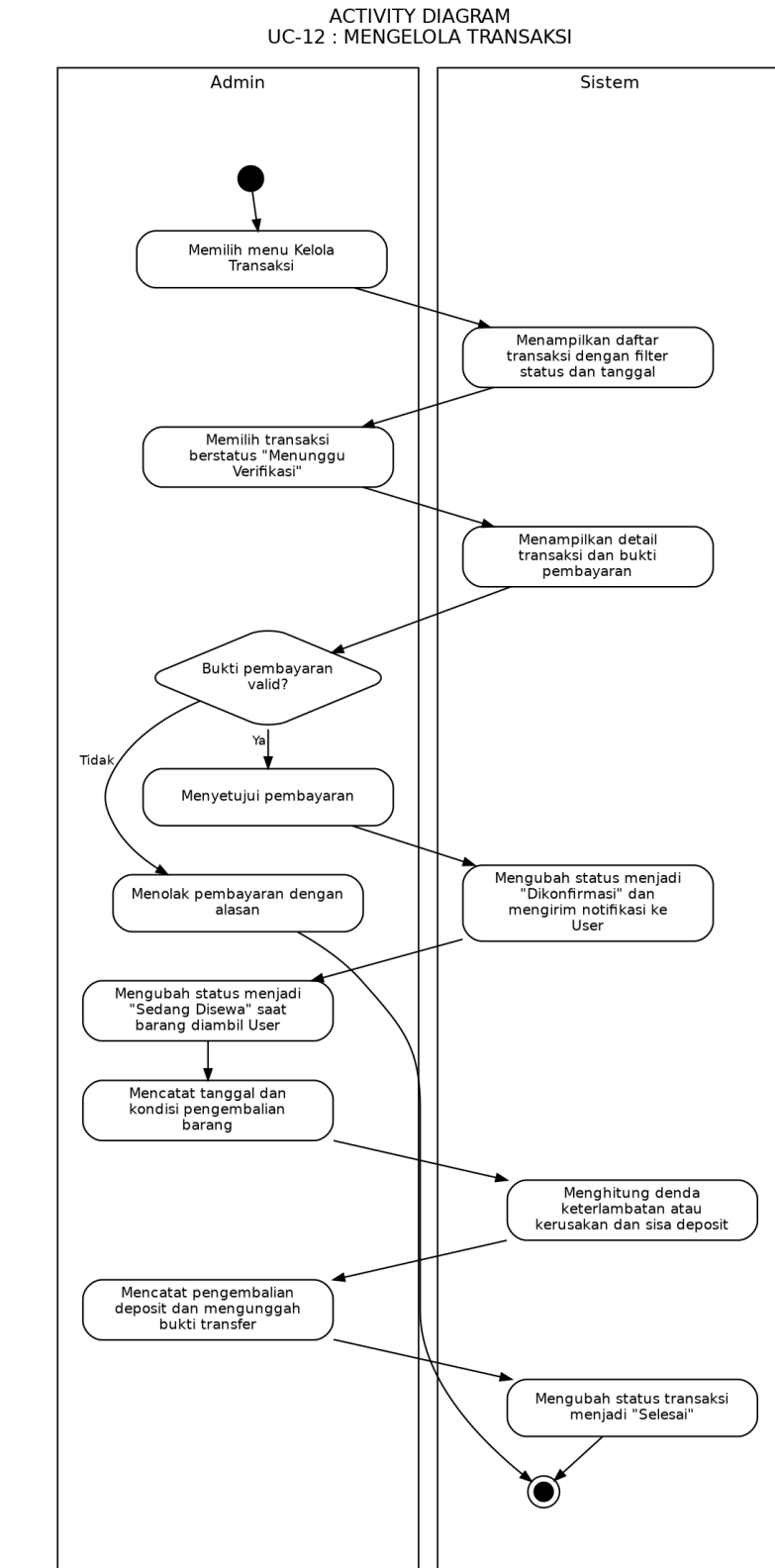
Gambar 3.40 Activity diagram #12 Mengelola Transaksi
