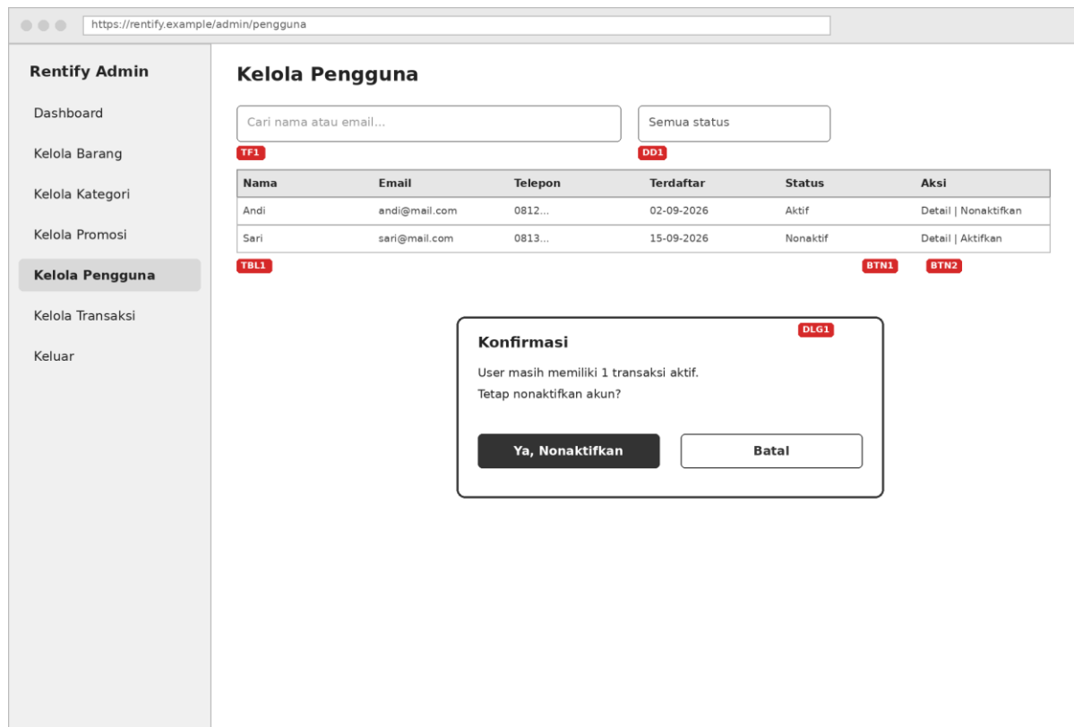
Gambar 3.34 Rancangan antarmuka P13 Kelola Pengguna
