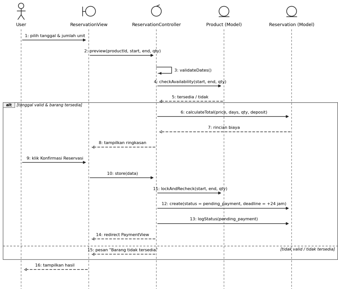
Gambar 3.18 Sequence diagram #6 Melakukan Reservasi
