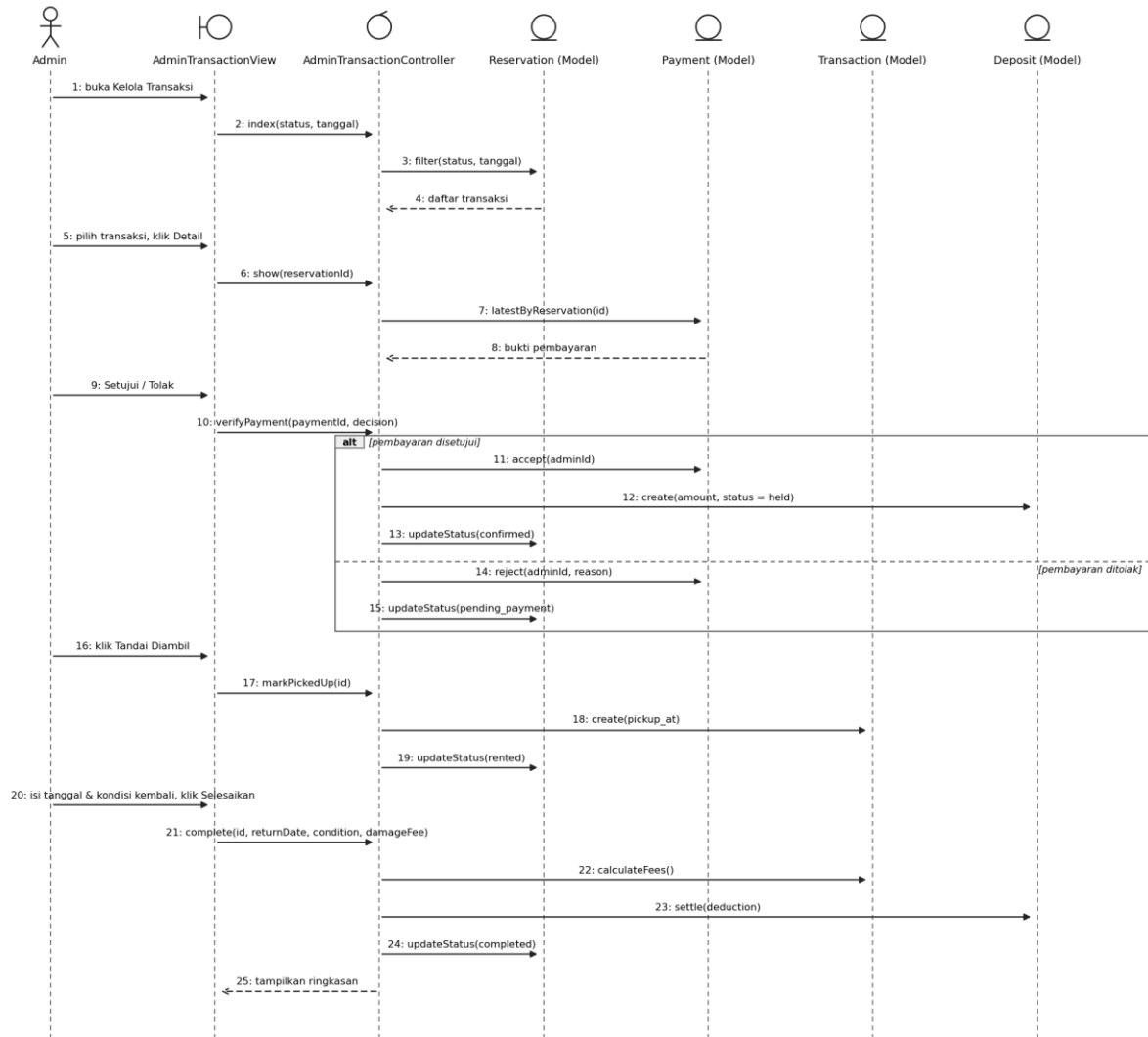
Gambar 3.39 Sequence diagram #12 Mengelola Transaksi
