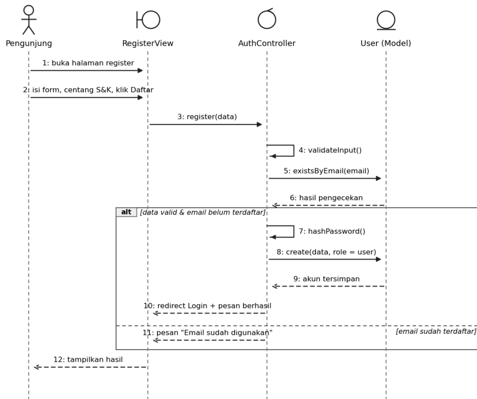
Gambar 3.6 Sequence diagram #2 Pendaftaran Akun
