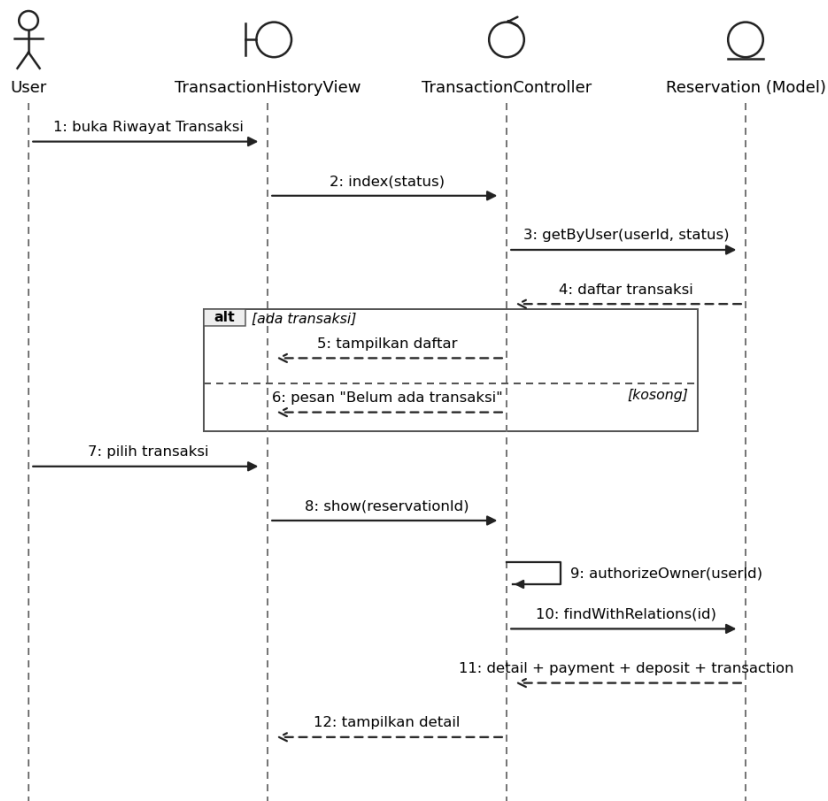
Gambar 3.24 Sequence diagram #8 Melihat Riwayat Transaksi
