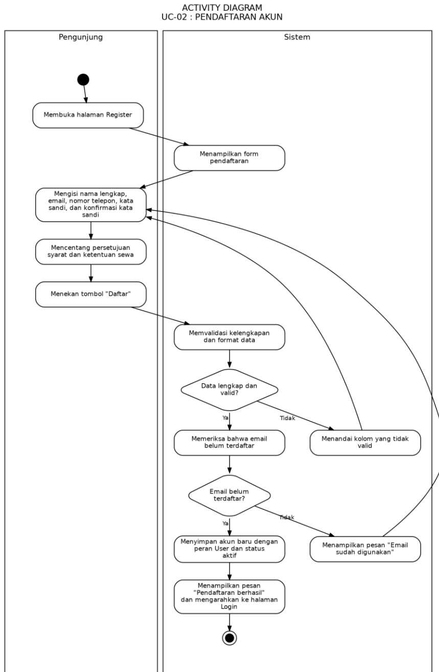
Gambar 3.7 Activity diagram #2 Pendaftaran Akun
