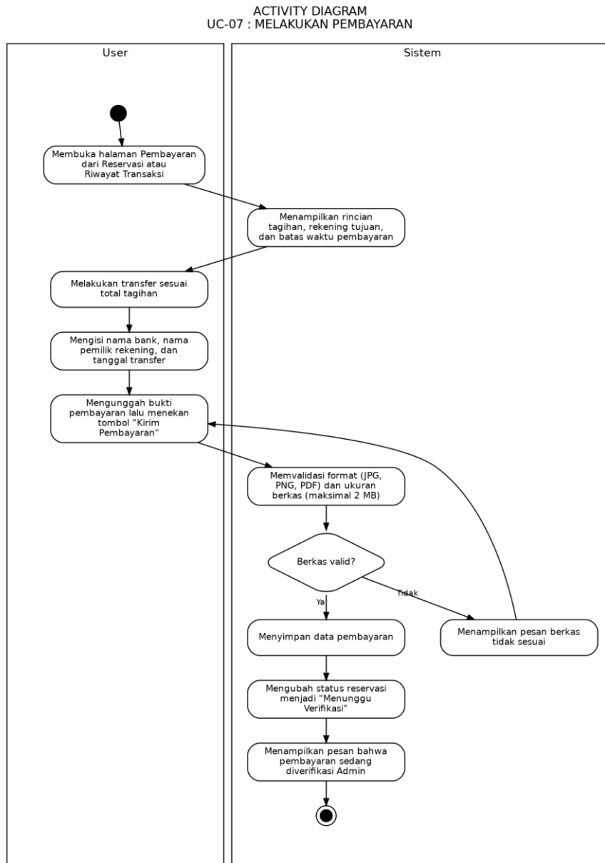
Gambar 3.22 Activity diagram #7 Melakukan Pembayaran
