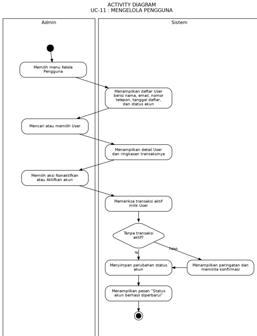
Gambar 3.36 Activity diagram #11 Mengelola Pengguna
