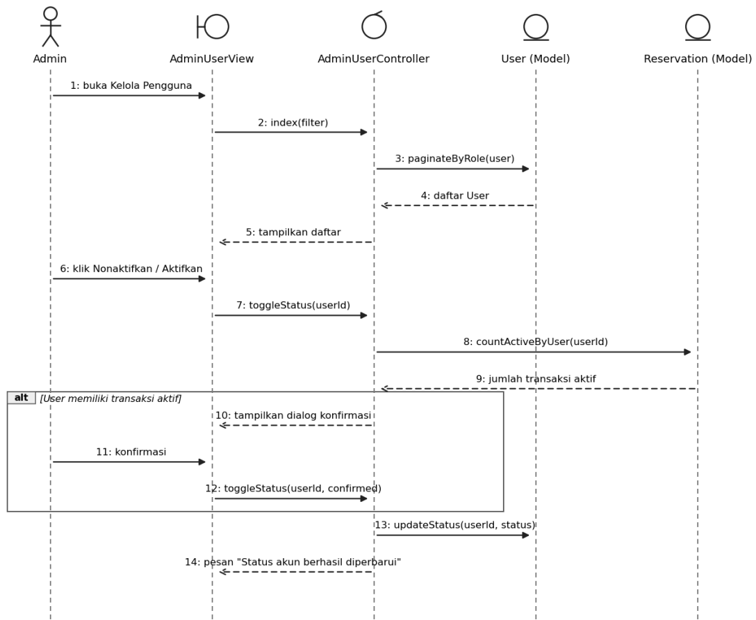
Gambar 3.35 Sequence diagram #11 Mengelola Pengguna
