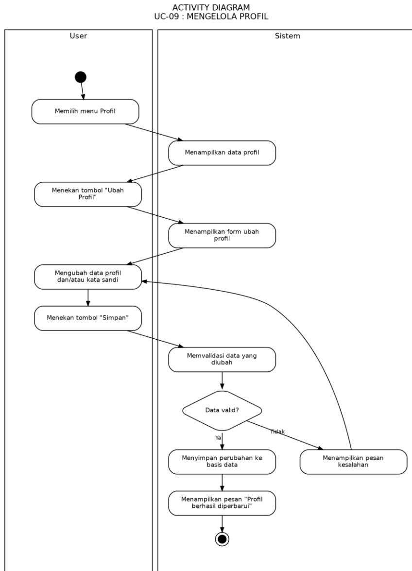
Gambar 3.28 Activity diagram #9 Mengelola Profil
