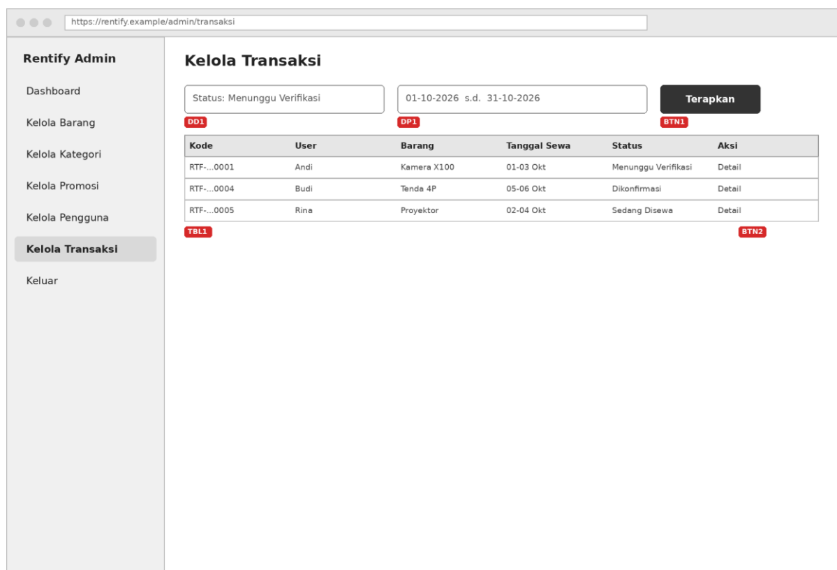
Gambar 3.37 Rancangan antarmuka P14 Kelola Transaksi
