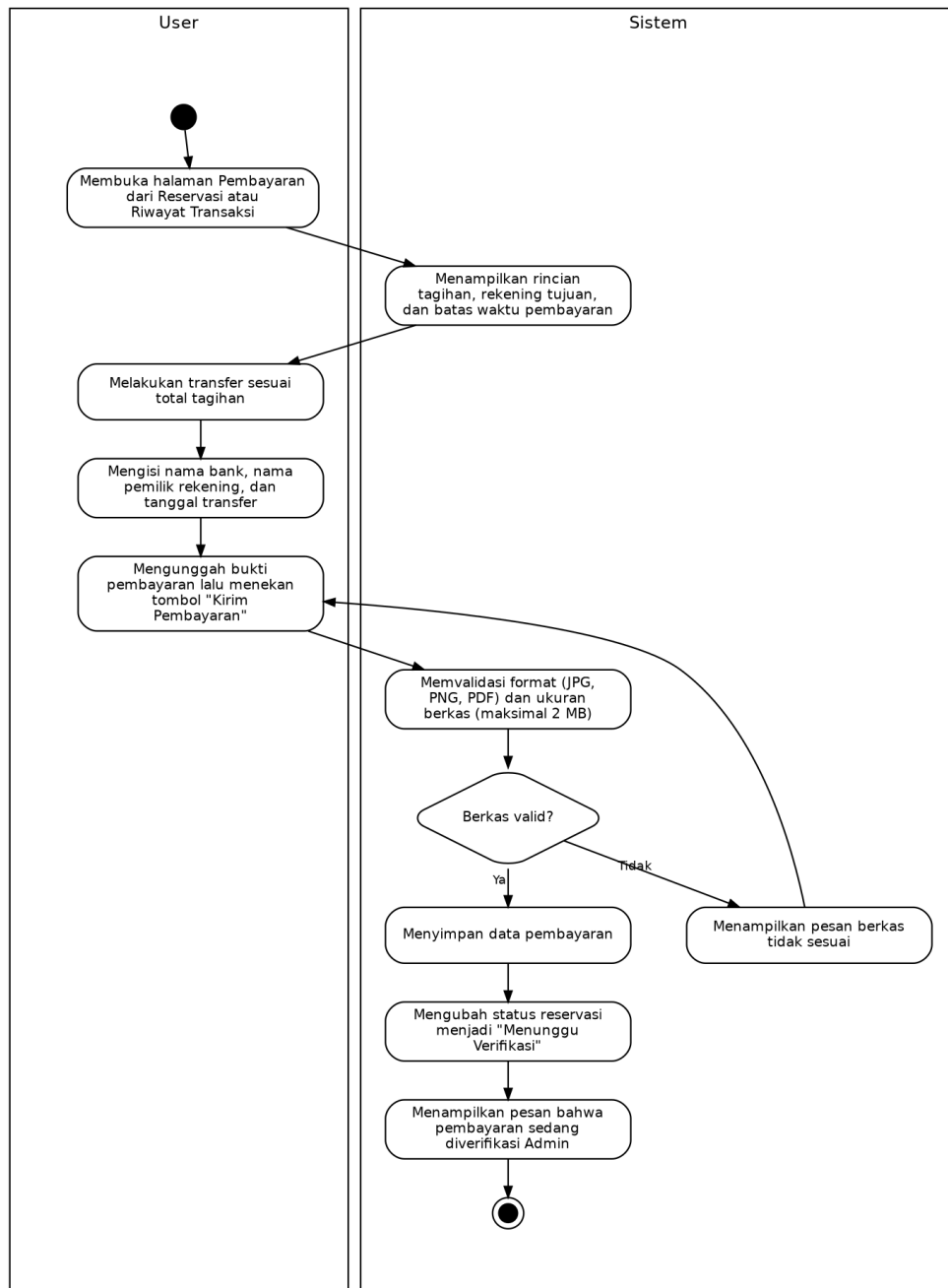
Gambar 3.9 Activity Diagram UC-07 Melakukan Pembayaran
