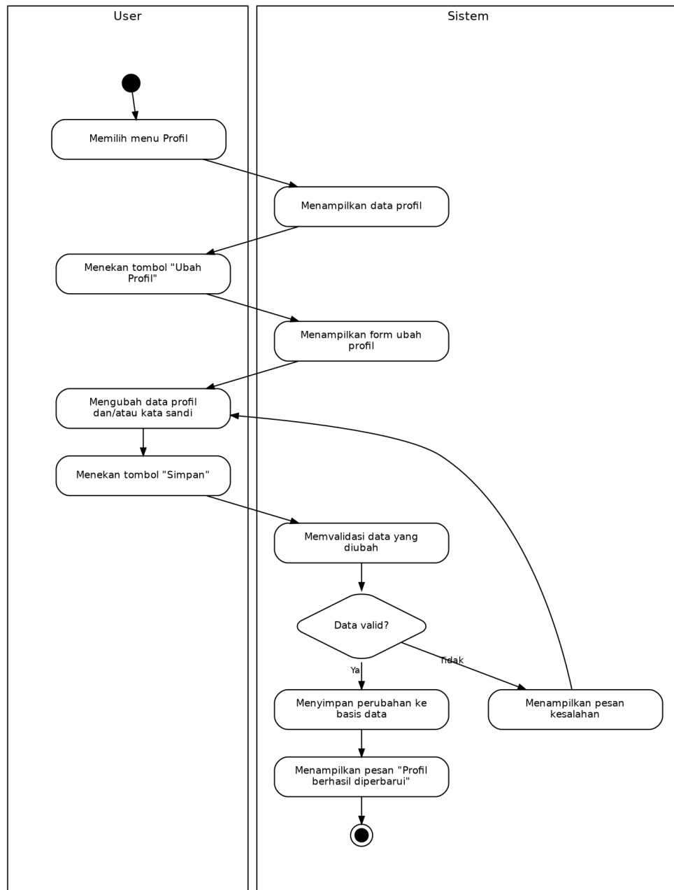
Gambar 3.11 Activity Diagram UC-09 Mengelola Profil
