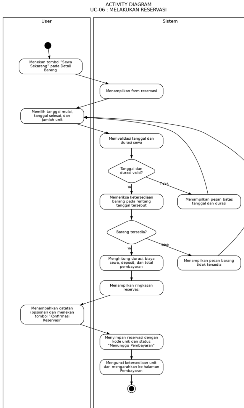
Gambar 3.8 Activity Diagram UC-06 Melakukan Reservasi
