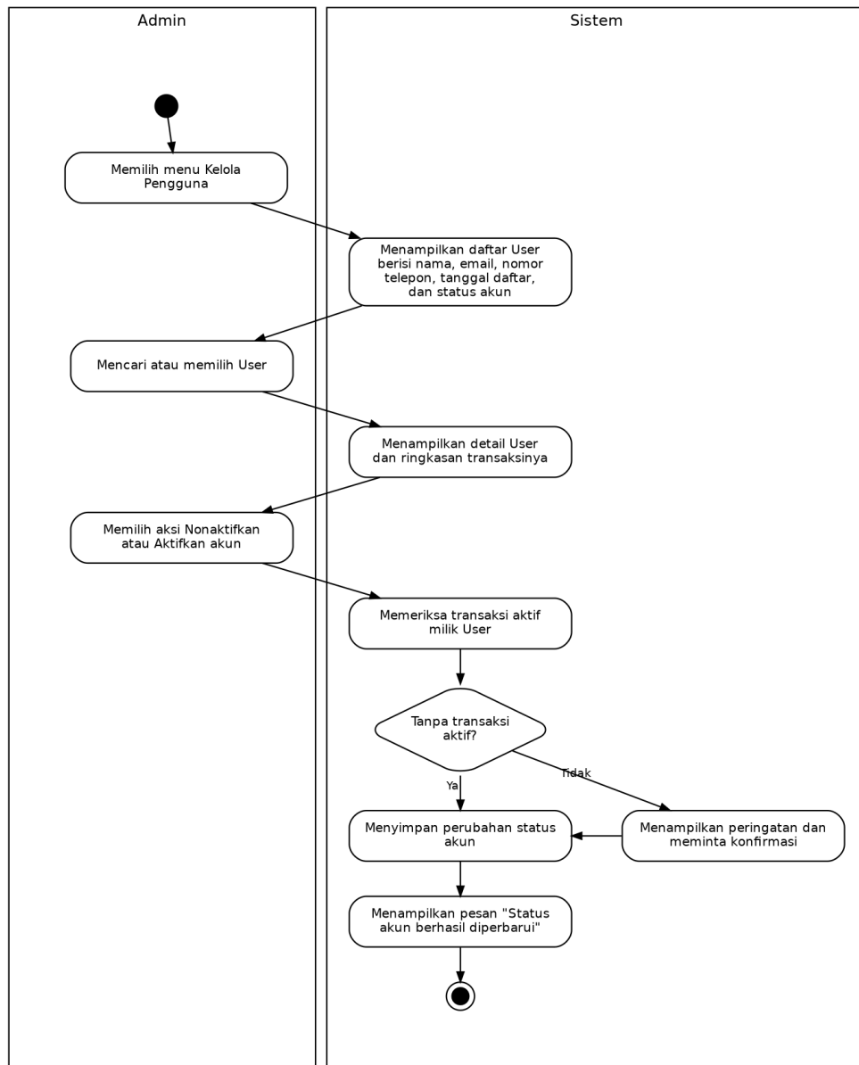
Gambar 3.13 Activity Diagram UC-11 Mengelola Pengguna
