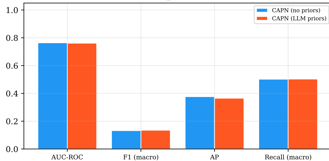
Capn Llm
