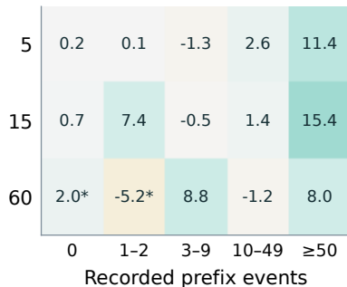
SEISMIC | QRF
