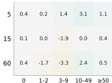
SEISMIC | NGBoost
