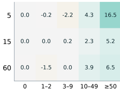
SEISMIC | QRF
