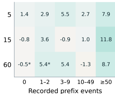
SEISMIC | NGBoost
