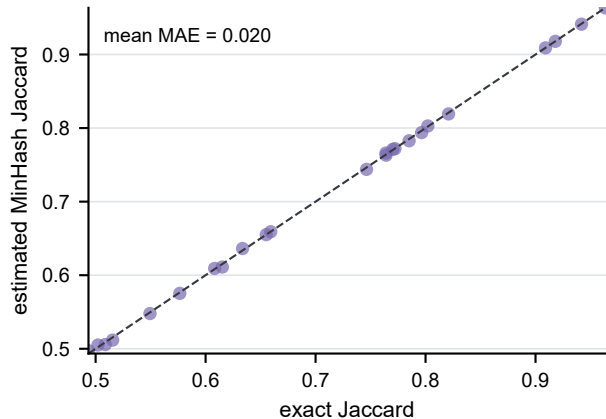
B. Native MinHash audit
