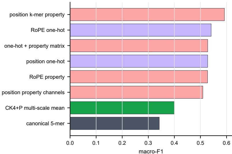
A. Motif-position readout
